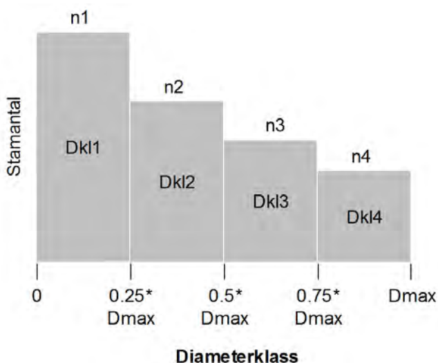
Figur 4.6. Diameterklasser för bedömning av fullskiktad skog.
