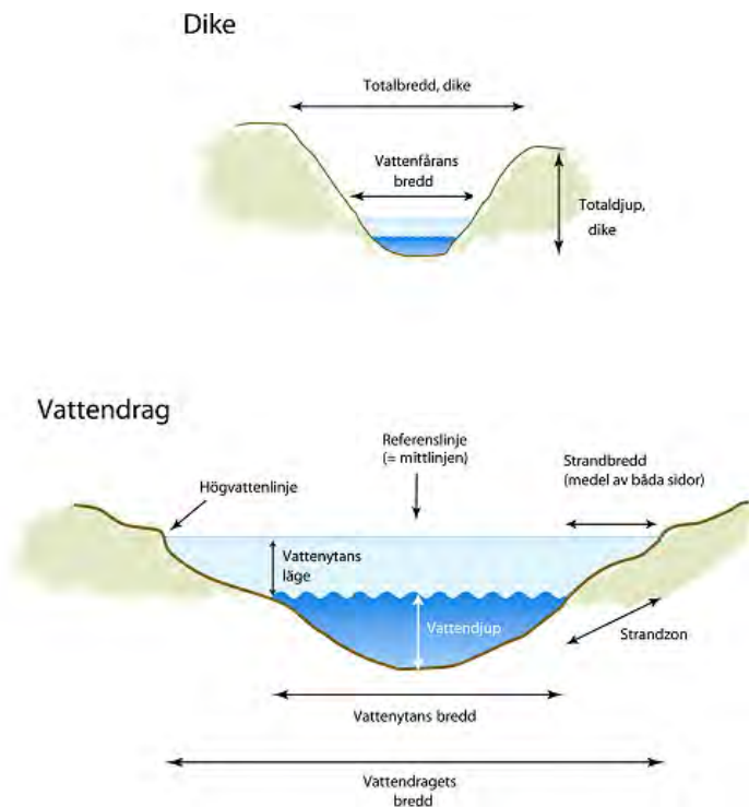
Figur 6.5. Beskrivning av referenslinjer och beskrivna zoner i diken och vattendrag.
