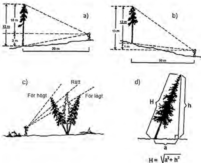
Figur B6. Höjdmätning med Suunto eller Silva höjdmätare.
