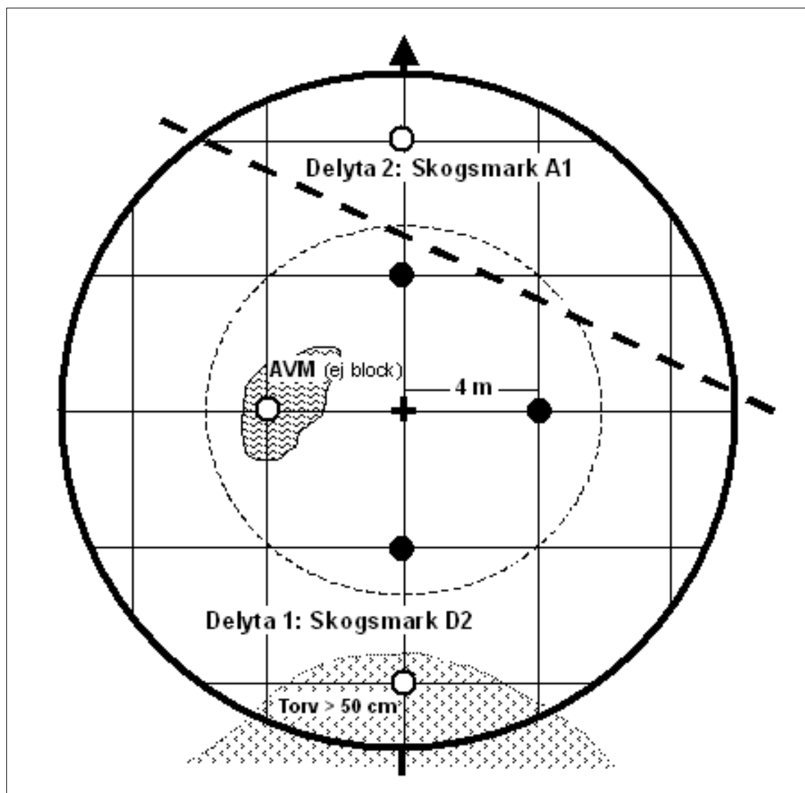
Fig. 5.1 Lägen på provytan (6 punkter) för sondering av sten och block. De tre svarta punkterna sondas. De tre vita punkterna sondas inte, då de ligger på ett torvlager > 50 cm, på AVM (exklusive block) samt på fel delyta.
