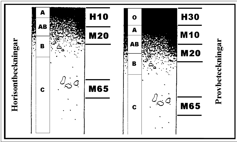
Fig. 11.7.24.6 Horisont- och provbeteckningar i profiler med respektive utan O-horisont.
