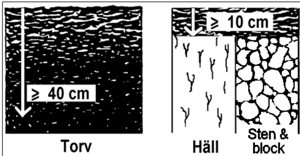
Fig. 11.7.24.1 För att klassificera Histosol ska organiskt material (H- eller O-horisont) finnas med minst 40 cm mäktighet, dock endast minst 10 cm mäktighet om skiktet ligger direkt på häll (eller sten och block).
