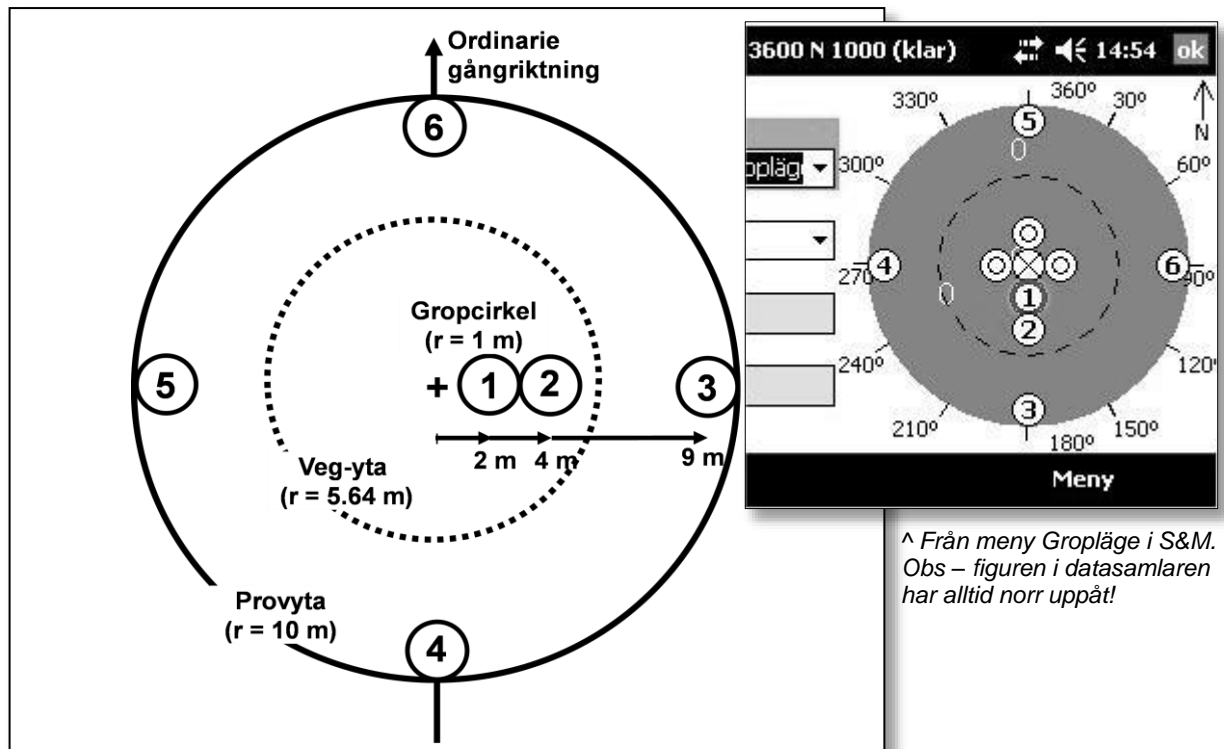
Fig. 11.3.1 Gropcirkelns fasta, alternativa lägen på provytan (gropläge 1-6).
