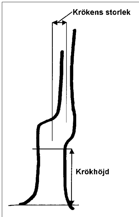
Fig. 8.5 Tvärkrök.
