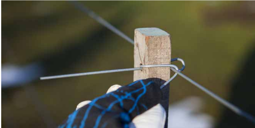
Bild 79 D. Böj clipset på vardera sidan stolpen på ovansidan om tråden.
