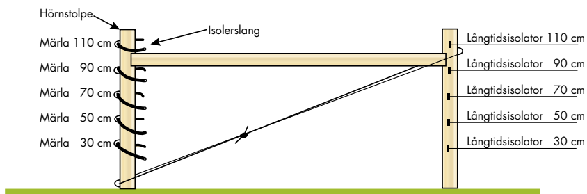
Bild 36. Skiss över parallellhörnets ena sida.
