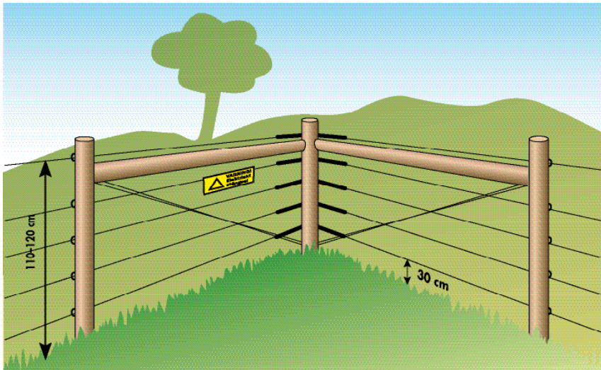
Bild 33. Parallellhörn med femtrådigt elstängsel.
