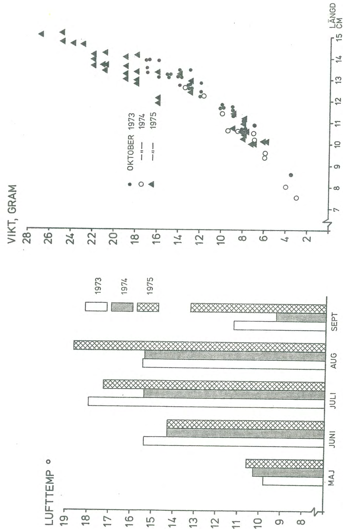
Fig. 11. Månadsmedeltemperatur (Vänersborg) och tillväxten hos gösungar i Dättern åren 1973-75.
