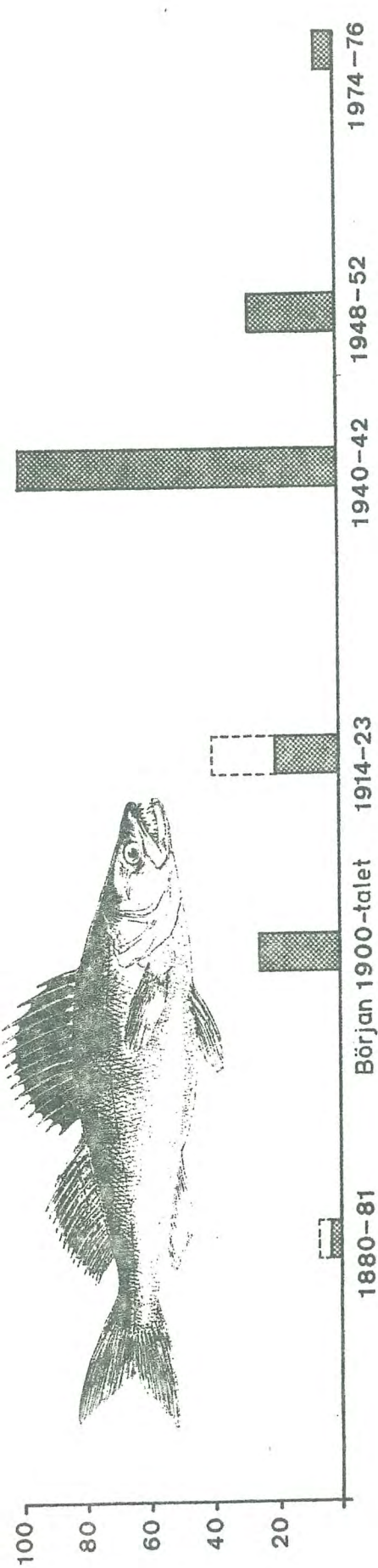
Fig. 10. Klimatet i Vänersborg och gösfångsten i Dättern.
