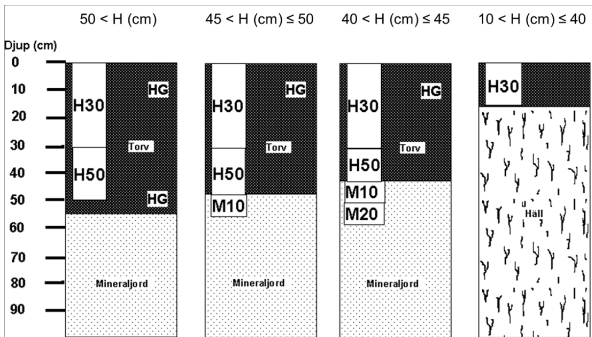
Fig. 11.7.24.2 Markprovtagning (H30-M20) och humifieringsgradsbestämning (HG) i några olika fall av Histosol.
