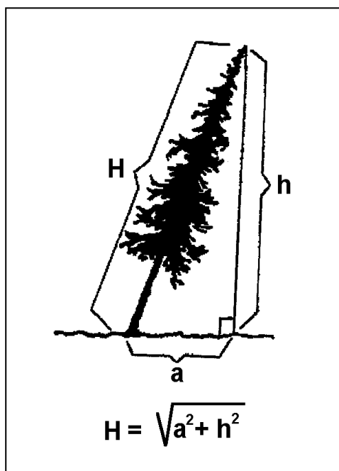
Fig. B1.2 Om trädet lutar starkt ( > 10^\circ ) mäts avståndet från marken till toppen ( h ). Därefter lodar man in den punkt som ligger rakt under trädets topp och mäter avståndet från denna till trädet ( a ). Trädets rätta höjd ( H ) beräknas som hypotenusan i en rätvinklig triangel, där kateterna ( a och h ) är kända.
