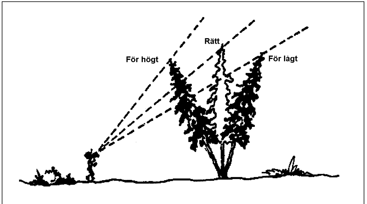
Fig. B1.1 Om trädet lutar mot den som mäter får man för högt mätvärde och om trädet lutar från den som mäter får man för lågt mätvärde.
