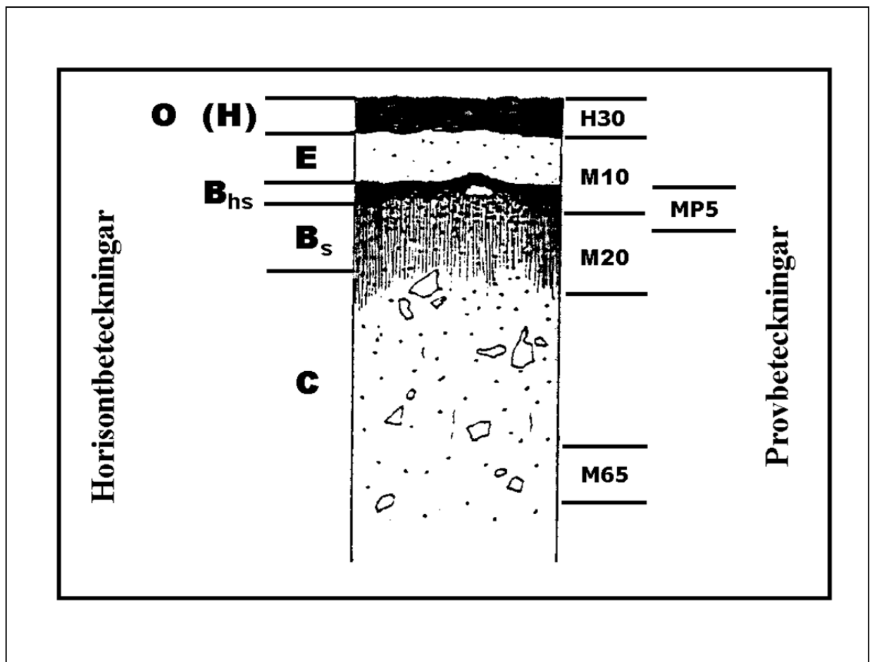
Fig. 11.7.24.5 Horisont- och provbeteckningar – Podzol.
