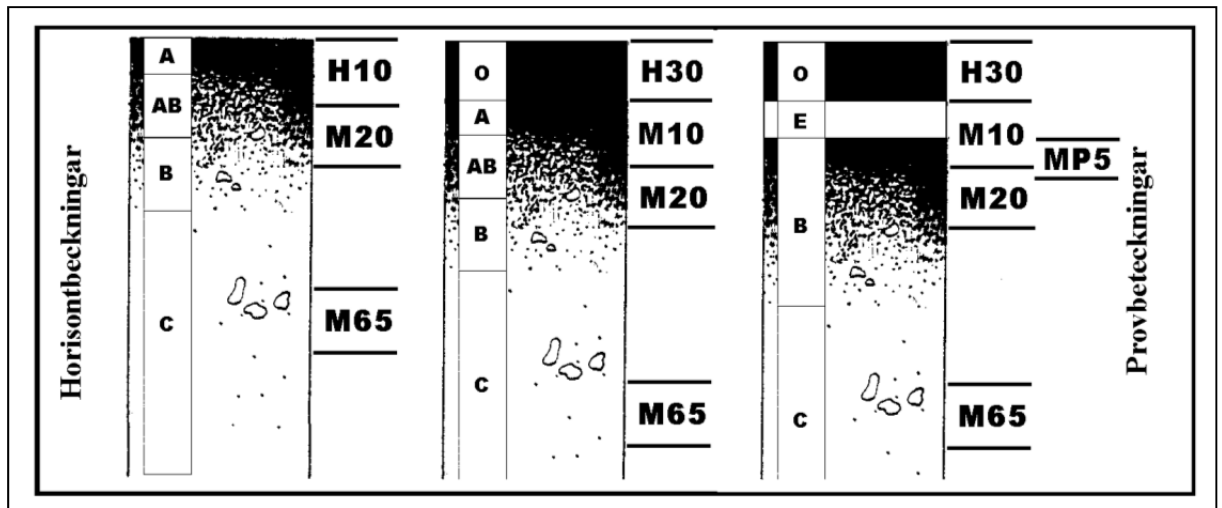
Fig. 11.7.24.6 Horisont- och provbeteckningar i profiler med respektive utan O-horisont, samt vid förekomst av E-horisont – Umbrisol, Arenosol, Cambisol och Regosol.
