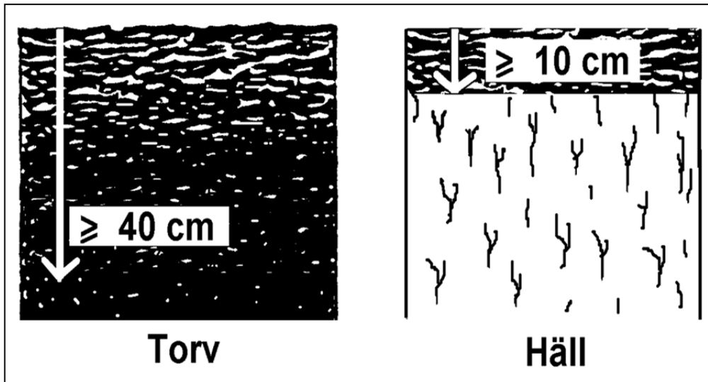
Fig. 11.7.24.1 För att klassificera Histosol ska organiskt material (H- eller O-horisont) finnas med minst 40 cm mäktighet, dock endast minst 10 cm mäktighet om skiktet ligger direkt på häll.
