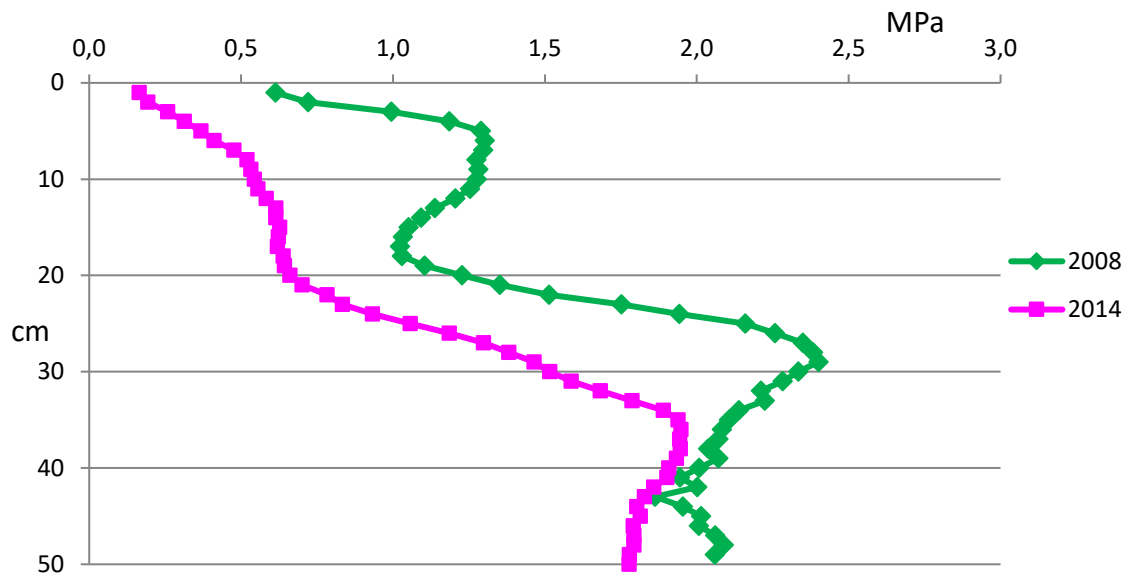
Figur 26. Penetrationsmotstånd i skiktet 0 - 50 cm, fält 26. Vattenhalten var 15 % (vikt-%) i skiktet 5 - 25 cm och 13 % (vikt-%) i skiktet 25 - 50 cm 2008 samt 16 % och 12 % 2014.
