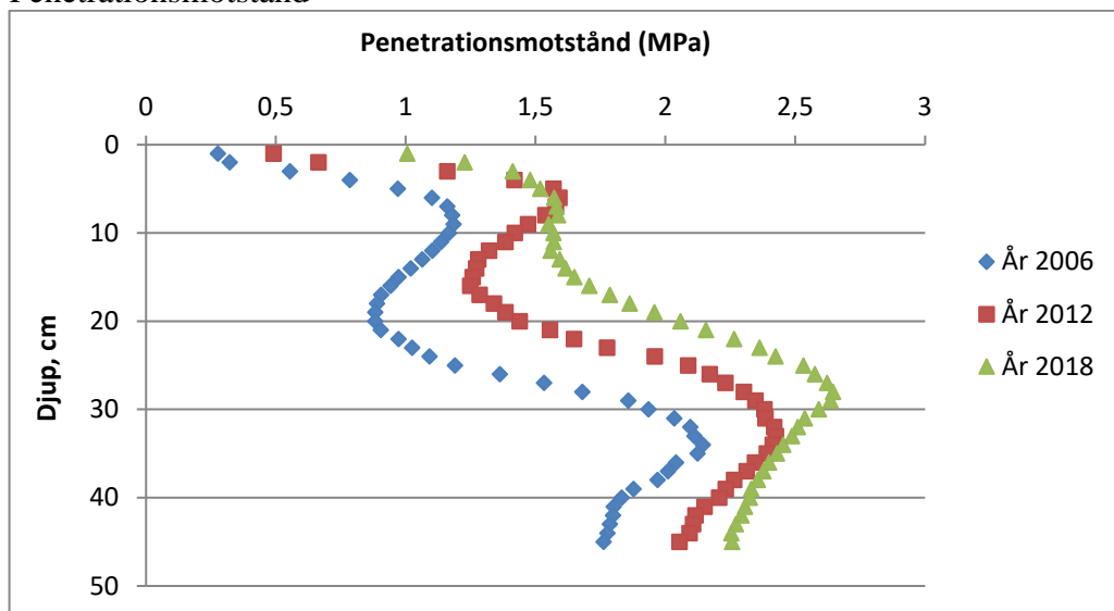
Figur 18. Penetrationsmotstånd i skiktet 0 - 50 cm, fält 18. Vattenhalten var 25 % (vikt-%) i skiktet 5 - 25 cm och 21 % (vikt-%) i skiktet 25 - 50 cm 2006, 18,8% och 17,0% 201 och 17,2 respektive 18,0 % år 2018.
