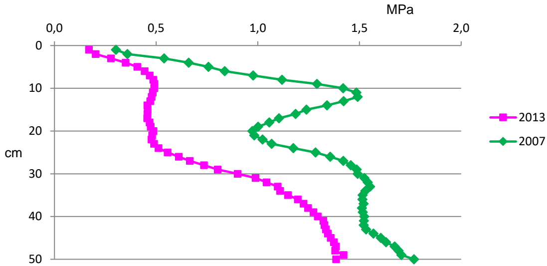
Figur 23. Penetrationsmotstånd i skiktet 0 - 50 cm, fält 23. Vattenhalten var 25 % (vikt-%) i skiktet 5 - 25 cm och 22 % (vikt-%) i skiktet 25 - 50 cm och 26 % respektive 25 % 2013.
