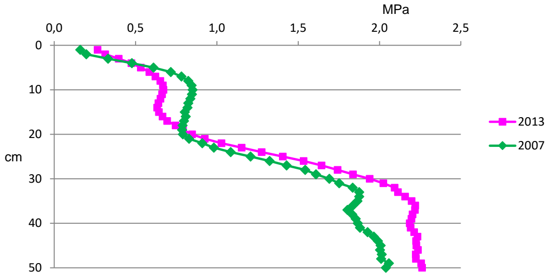
Figur 21. Penetrationsmotstånd i skiktet 0 - 50 cm, fält 21. Vattenhalten var 20 % (vikt-%) i skiktet 5 - 25 cm och 24 % (vikt-%) i skiktet 25 - 50 cm 2007 och 23 % respektive 17 % 2013.
