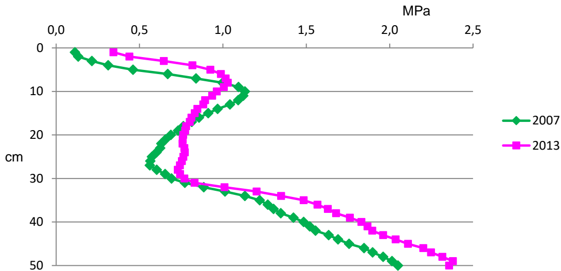
Figur 24. Penetrationsmotstånd i skiktet 0 - 50 cm, fält 24. Vattenhalten var 24 % (vikt-%) i skiktet 5 - 25 cm och 18 % (vikt-%) i skiktet 25 - 50 cm och 19 % respektive 18 % 2013.
