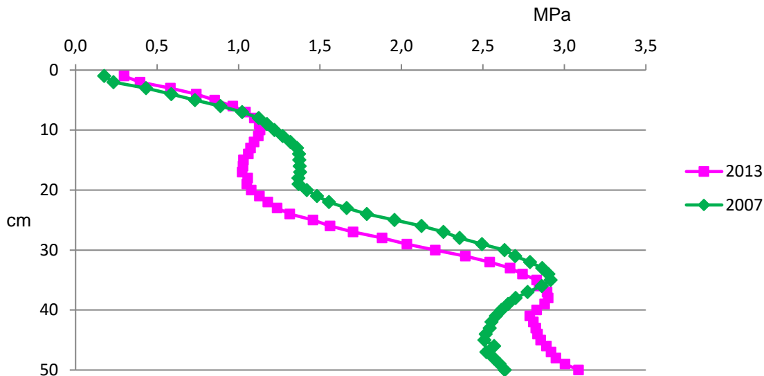
Figur 22. Penetrationsmotstånd i skiktet 0 - 50 cm, fält 22. Vattenhalten var 21 % (vikt-%) i skiktet 5 - 25 cm och 17 % (vikt-%) i skiktet 25 - 50 cm och 21 % respektive 17 % 2013.
