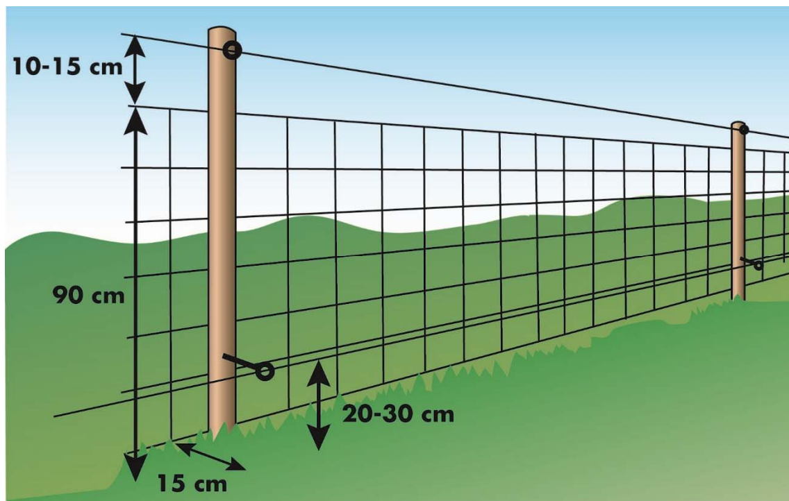
Figur 6. Skiss av fårnät kompletterat med två eltrådar. Bilden är lånad från Viltskadecenter.
