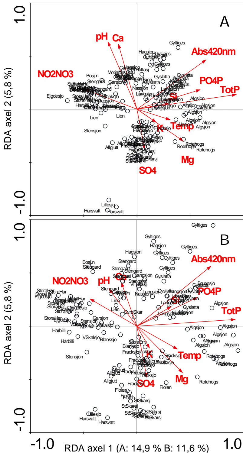
Figur 5. RDA diagram som visar vilken kombination av miljövariabler som samvarierar med växtplanktons samhällsstruktur i sjöarna. Diagram A visar sambandet om man analyserar årsmedelvärden för de 29 sjöarna baserat på sju provtagningar per år, där miljövariablerna förklarar 35 % av variationen hos växtplankton. Diagram B visar motsvarande samband baserat på årsmedelvärden för fyra provtagningar per år, där miljövariablerna förklarar 31 % av variationen hos växtplankton. Antalet provtagningspunkter är 113 i båda diagrammen. Värden inom parentes för axlarna visar förklaringsgraden.
