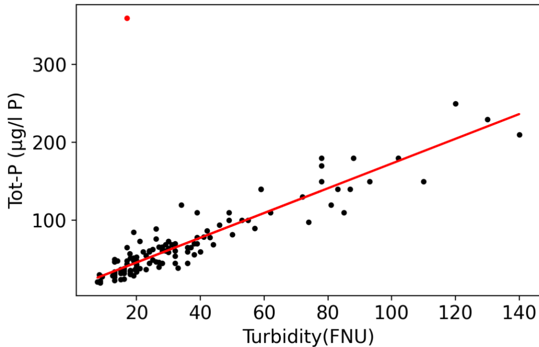
Figur 2: Regression mellan turbiditet och TotP i Lärjeån. Data från recipientkontrollen (2012–2025).
