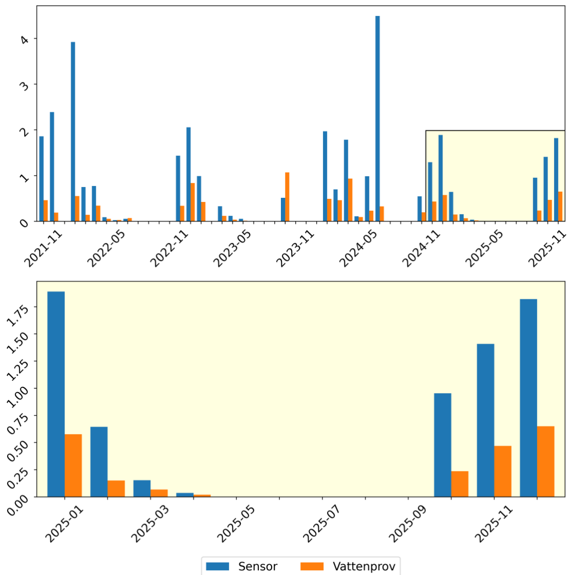
Figur 7: Månadstransporter av fosfor i Lärjeån beräknat från dygnsmedelvärden av turbiditet samt månadsvisa uppmätta halter av TotP (ton).
