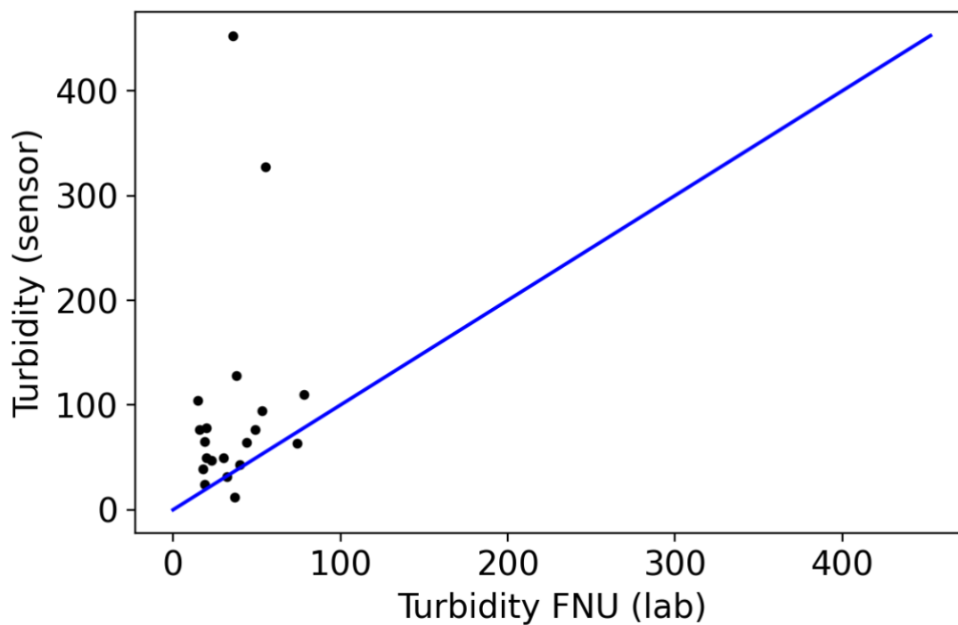
Figur 1: Dygnsmedelvärden av turbiditet från sensor (y-axel) jämförd med turbiditet från labanalyserade vattenprover (x-axel) från åren 2021–2025. Den blå linjen avser 1:1 linjen.
