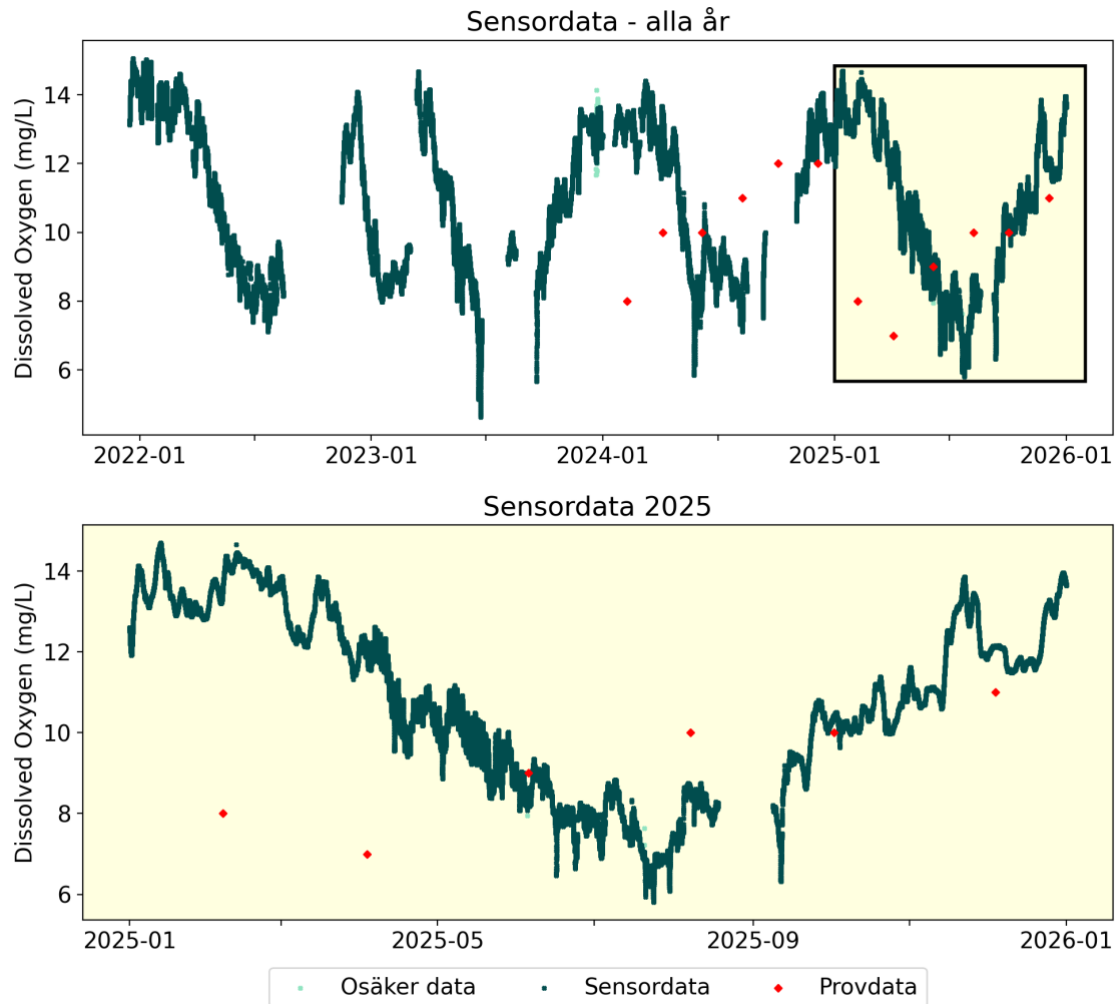
Figur 6: Tidsserie av syre i Lärjeån med sensordata var 15:e minut. De ljusare partierna representerar tveksamma mätvärden.
