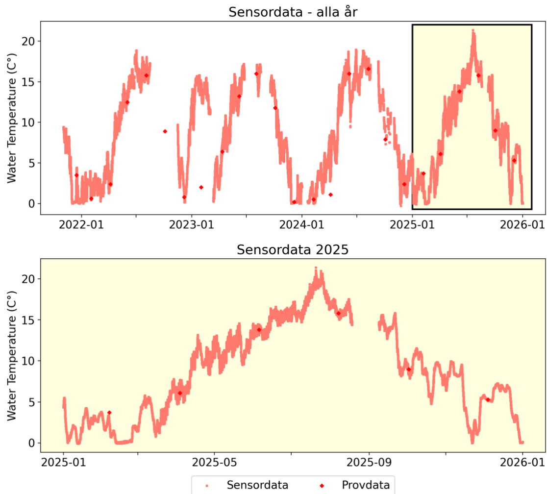
Figur 5: Tidsserie av temperaturen i Lärjeån med sensordata var 15:e minut (orange), observerade temperaturvärden är markerade med röda punkter.
