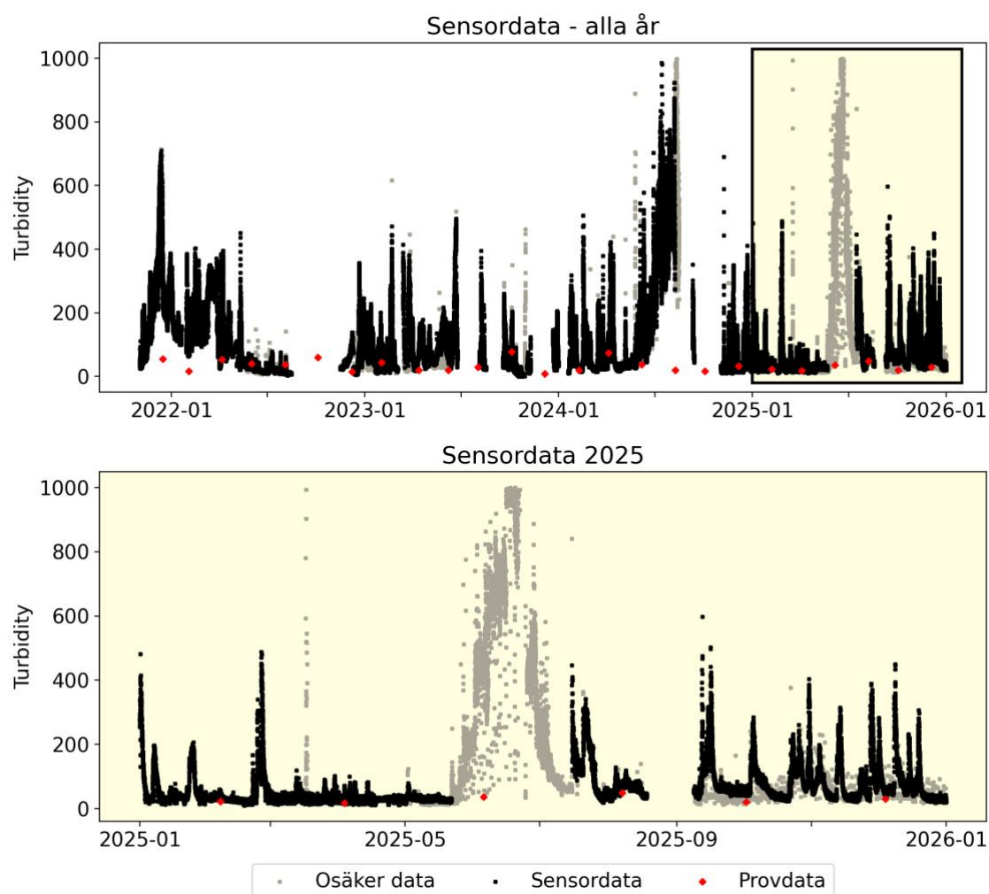
Figur 3: Tidsserie av turbiditeten i Lärjeån med sensordata var 15:e minut (svart) samt månadsvisa vattenprover (röd). De ljusare partierna representerar tveksamma mätvärden. (Dessa har exkluderats från transportberäkningarna nedan).
