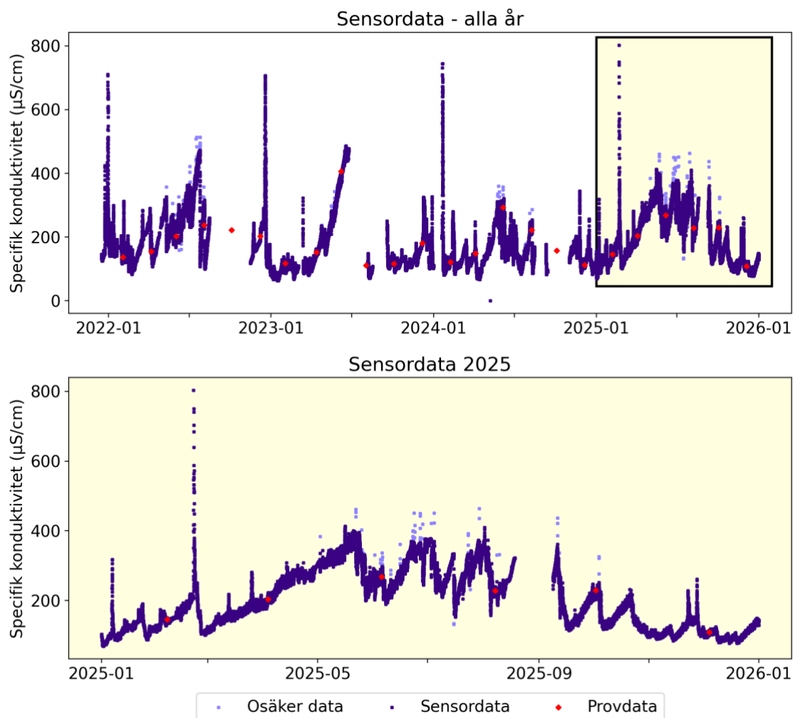
Figur 4: Tidsserie av konduktiviteten i Lärjeån med sensordata var 15:e minut. De ljusare partierna representerar tveksamma mätvärden.
