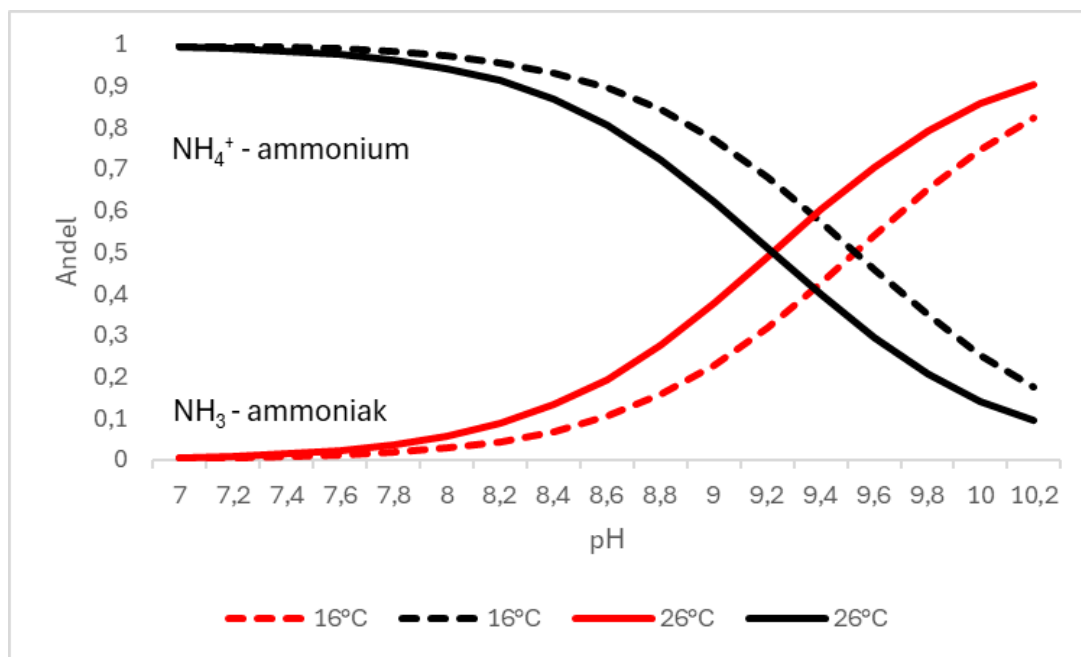
Figur 3. Figuren visar förhållandet mellan pH och temperatur på NH 3 /NH 4 + förhållandet i sötvatten.
