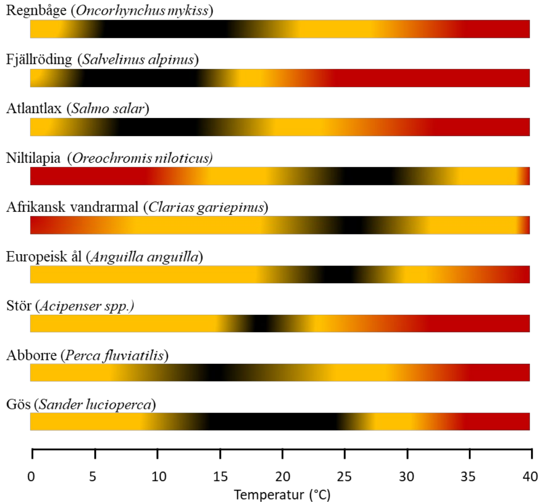
Figur 2. Rekommenderade (svart), tolererade (gult) och dödliga (rött) miljöförhållanden för fiskarter som förekommer i svenskt vattenbruk. Värdena baseras på publicerade källor (Thorpe, 1977; Sadler, 1979; Britz & Hecht, 1987; Lehtonen, 1996; Pyka & Kolman, 2003; Frisk et al., 2012; Sandblom et al., 2016; Castellano et al., 2017; Ogunji & Awoke, 2017; Yang et al., 2021; Korus et al., 2024, samt de referenser som nämns i texten ovan) och ska betraktas som generella riktlinjer. De kan variera beroende på art, livsstadium, andra vattenkvalitetsparametrar och lokala uppfödningförhållanden. Intervallen ovan är inte "skarpa gränsvärden" utan riktvärden för stabil drift. Snabba förändringar (även inom toleransområdena) kan vara stressande och bör undvikas.
