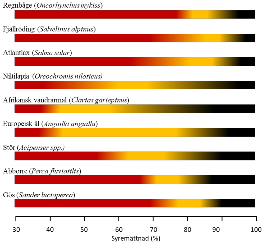
Figur 6. Rekommenderade (svart), tolererade (gult) och dödliga (rött) miljöförhållanden för fiskarter som förekommer i svenskt vattenbruk. Värdena baseras på publicerade källor (Alabaster et al., 1957; Wedemeyer, 1996; Tesch & Thorpe, 2003; Molleda et al., 2007; Olele & Tighiri, 2010; Chebanov et al., 2011; Woynarovich et al., 2011; Boyd & Tucker, 2012; Remen et al., 2012; Kestemont et al., 2015; Pedrazzani et al., 2020) och ska betraktas som generella riktlinjer. De kan variera beroende på art, livsstadium och lokala uppfödningförhållanden. Intervallen ovan är inte "skarpa gränsvärden" utan riktvärden för stabil drift. Snabba förändringar (även inom toleransområdena) kan vara stressande och bör undvikas.
