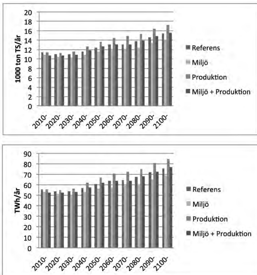
Figur 4.2 Årlig bruttomängd skogsbränsle i form av grot (grenar, toppar & barr) från gallring och slutavverkning enligt fyra scenarier återgivet i ton torr biomassa (övre) och energimängd (nedre). Observera att det är den fysiskt tillgängliga mängden i skogen som anges och inte den på marknaden realiserade mängden. Baserad på SKA-VB 08, SLU (Skogsstyrelsen 2008c).
