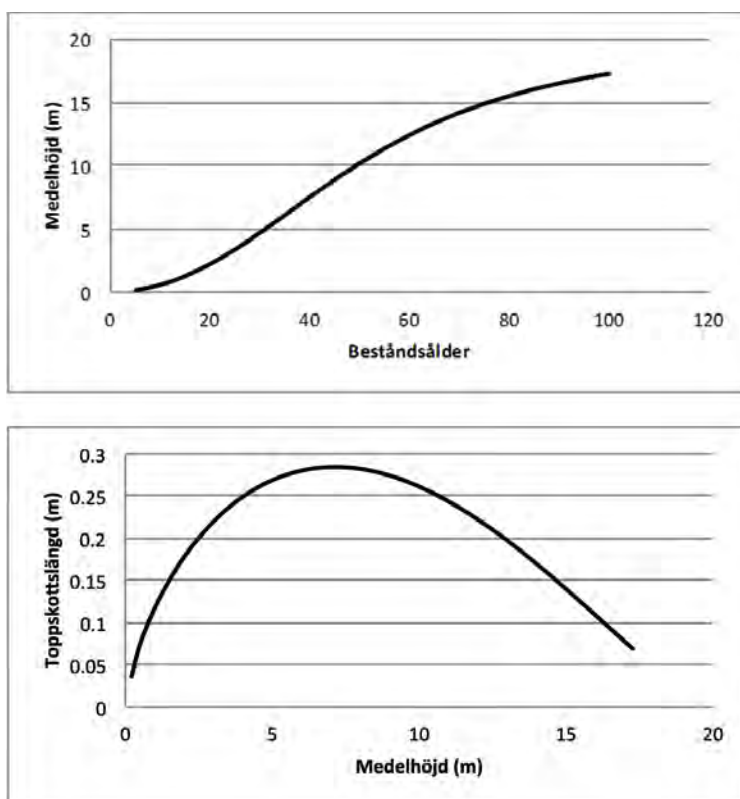
Figur 4.6 Den övre figuren visar medelhöjdens förväntade utveckling för granar på en mark med ståndortsindex G20 och den nedre visar förväntad toppskottslängd för en gran på samma mark vid given trädhöjd (Elfving 1982).
