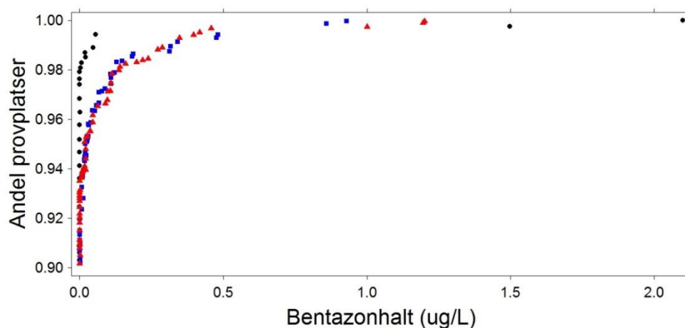
Figur 6. Sannolikhetsfördelningar för bentazonhalter i svenskt grundvatten uppdelad i tre klasser med avseende på andel åkermark i kommunen (svarta cirklar < 15 %, blåa fyrkanter 15-30 %, röda trianglar > 30 %). Kurvorna visar andel provplatser (y-axeln) där bentazonhalten i grundvatten understiger det angivna värdet på x-axeln.
