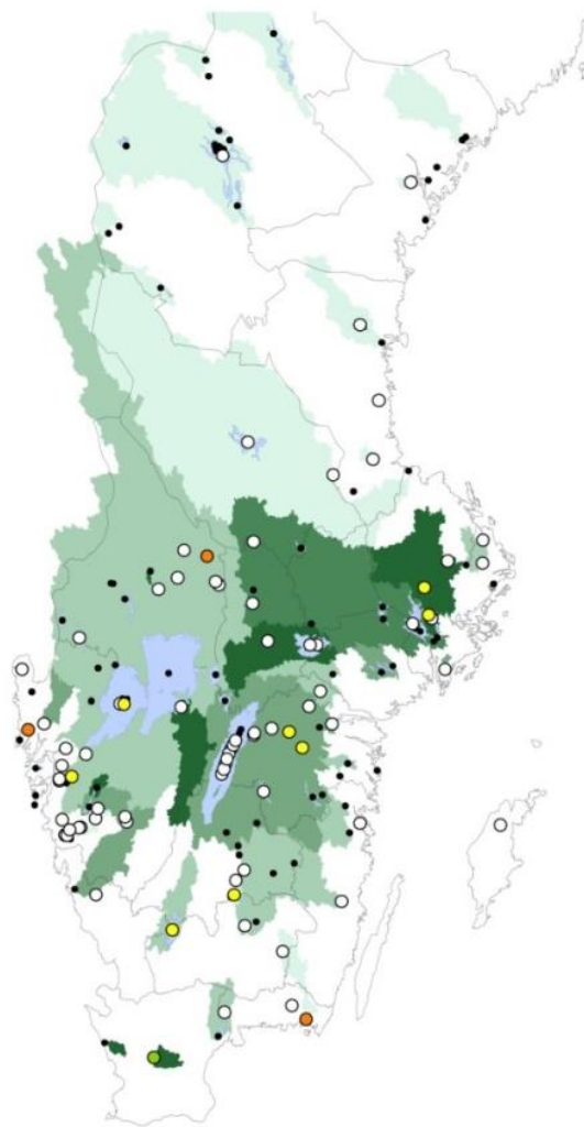
Figur 7. Resultat för provtagningsplatser i SGU:s vattentäcksarkiv tillsammans med andel åkermark i avrinningsområdet.
