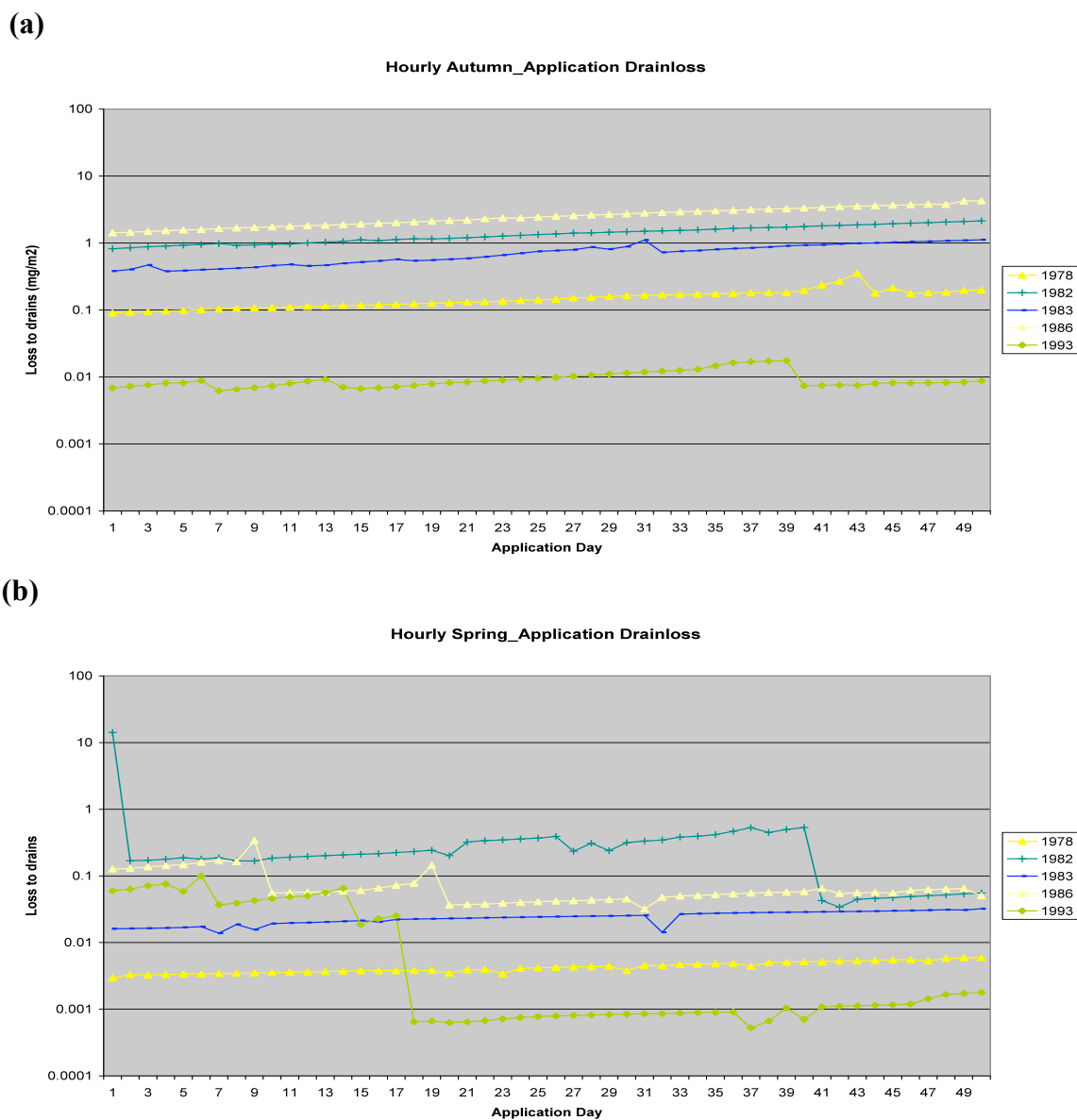
Figur 4. Total förlust via dräneringsvatten av typisk herbicid ( \text{mg/m}^2 ), för 50 spridningstidpunkter, under fem olika år: (a) Höstspridning; (b) Vårspridning. (Data från Lewan et al., 2009).
