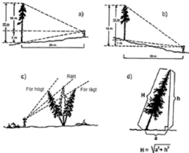
Figur B7. Höjdmätning med Suunto eller Silva höjdmätare.
