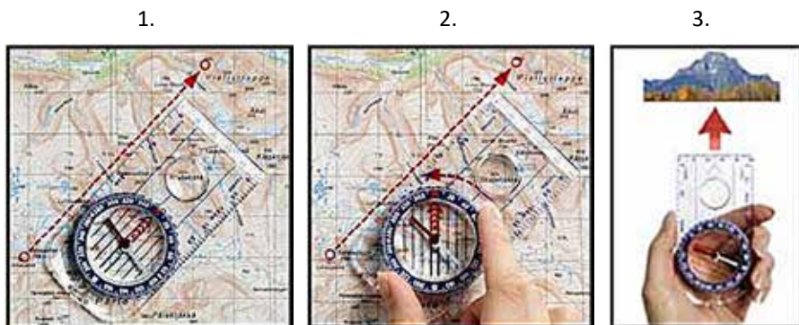
Figur B11. Navigering med kompass.
