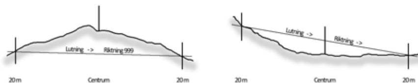
Figur 6.8. Mätning av marklutning.
