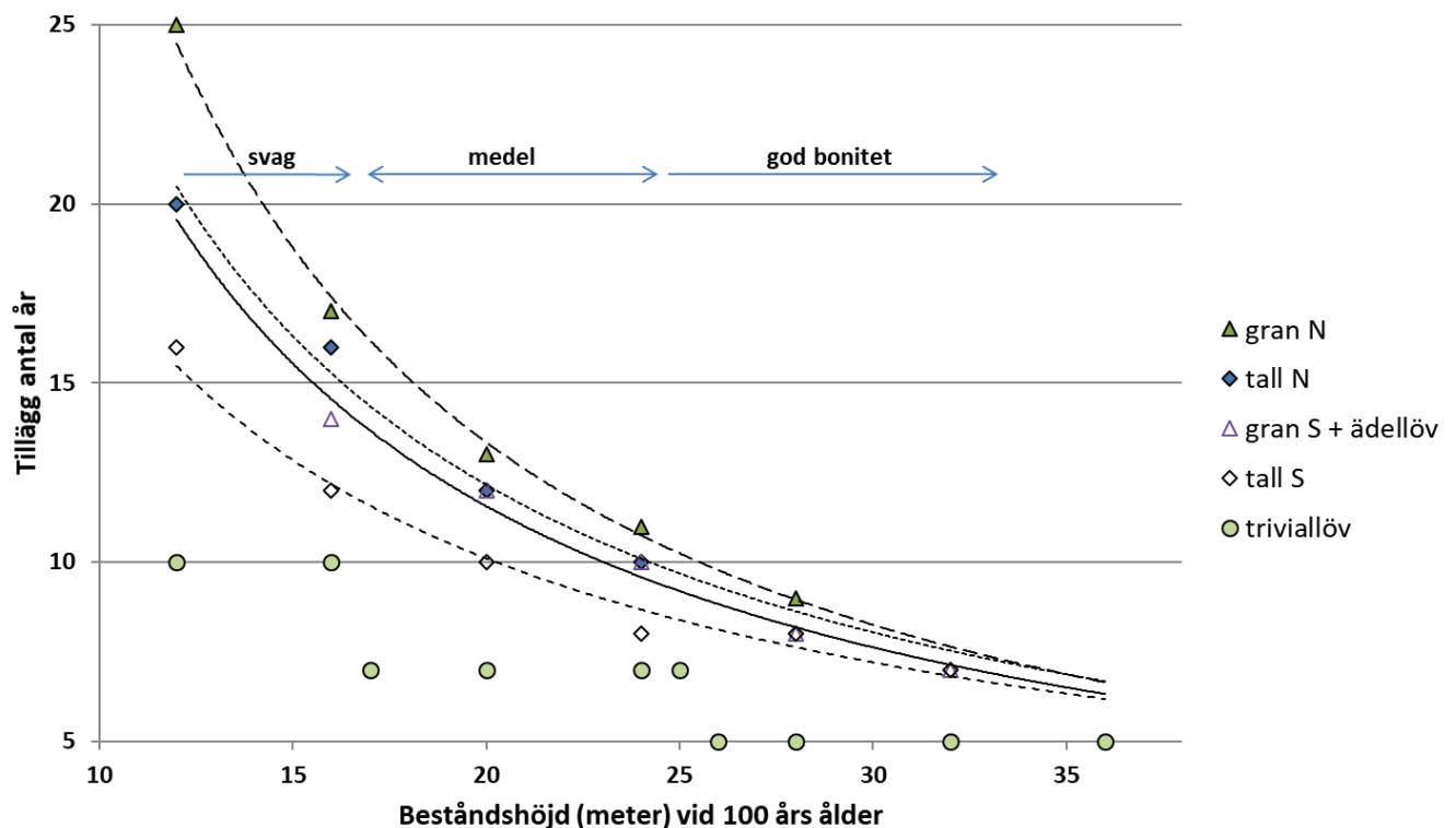
Figur 8. Antal år som det har tagit för beståndet att nå brösthöjd i förhållande till beståndshöjd och trädslag. Figuren är modifierad variant av figur 3 i Gardfjell och Hagner (2019).
