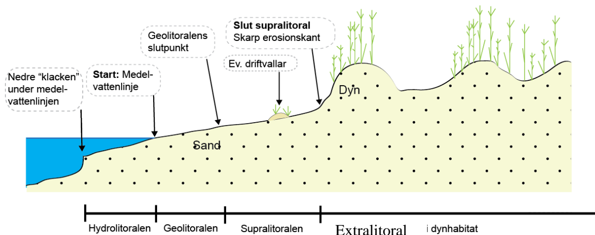
Figur 3. Sandstrand som övergår i dynamråde i profil. För detaljer om transektens fortsättning i extralitoralerna se 3.8.3. Detaljerad uppdelning av dynhabitat (2100) och figur 6.
