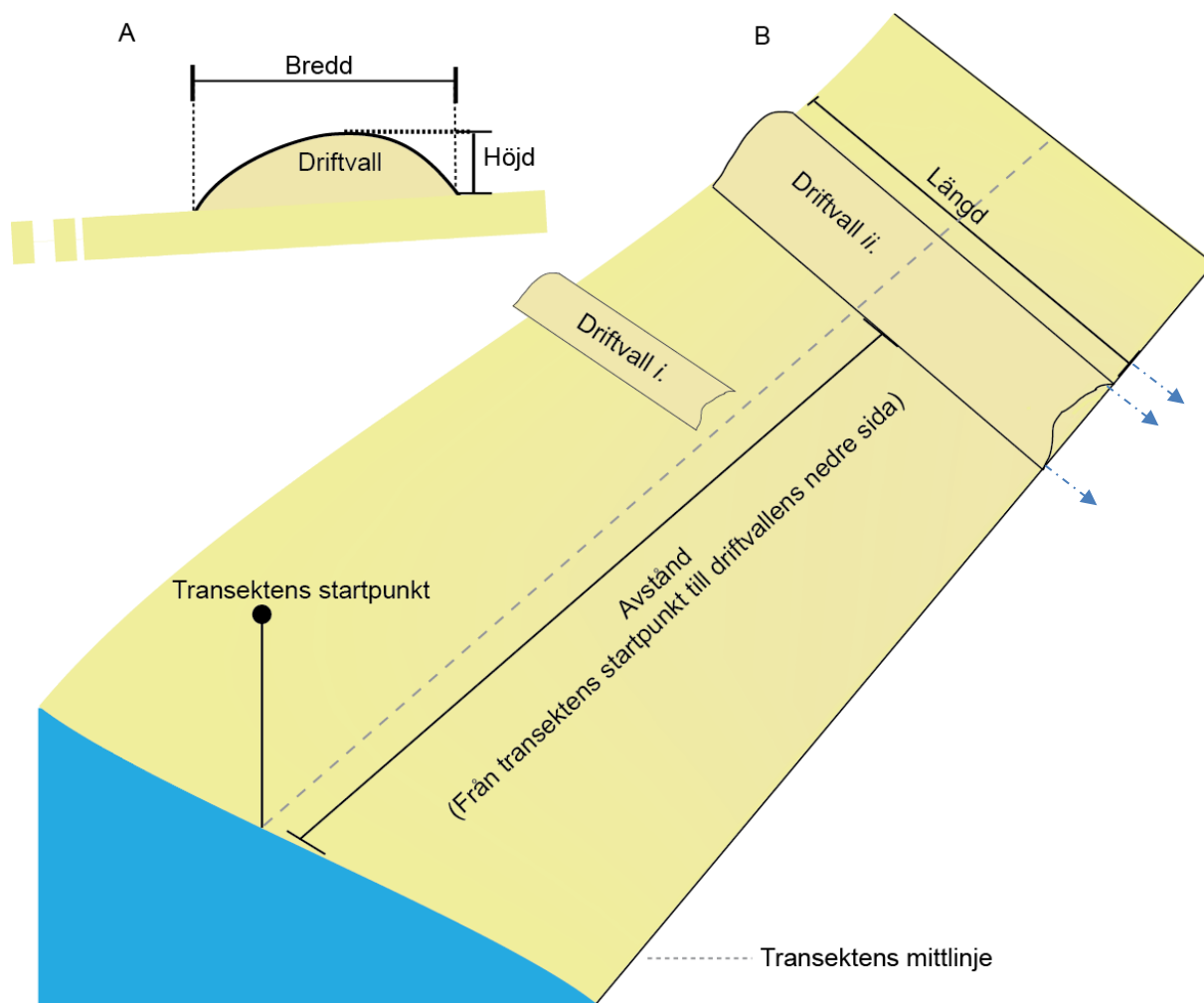
Figur 4. Driftvall. A, visar hur driftvallens höjd och bredd mäts. B, visar hur avstånd och längd mäts. Driftvall i. noteras inte i protokollet eftersom den inte skärs av transectens mittlinje. Driftvall ii. skärs av mittlinjen och noteras därmed i protokollet.
