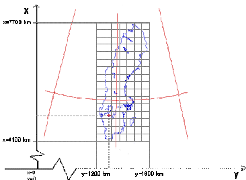
Figur B11. Plant koordinatsystem med medelmeridianens bild som x-axel.
