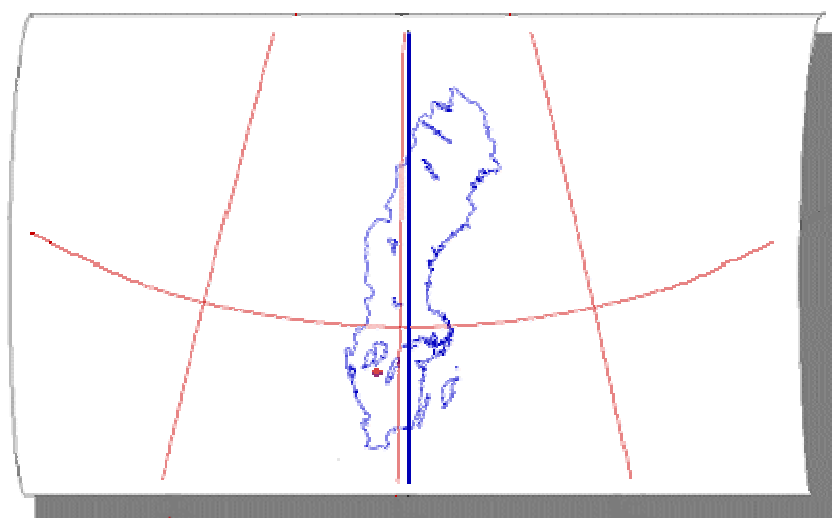
Figur B10. Medelmeridianen för Sverige och konvergerande meridianer.
