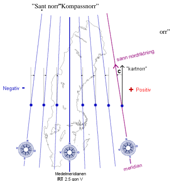
Figur B14. Meridiankonvergens i Sverige med de vinklar som man kan behöva justera för när man ska korrigera kompassens missvisning. Modifierad figur från lantmäteriets hemsida, med inlagda vinklar och riktningar.
