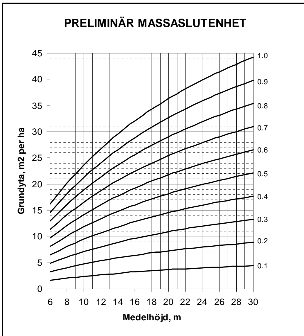
Figur B5. Diagram för bedömning av massaslutenhet
