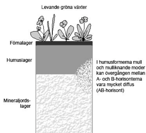
Figur 4.7. Jordprofil där olika lager och skikt illustreras.
