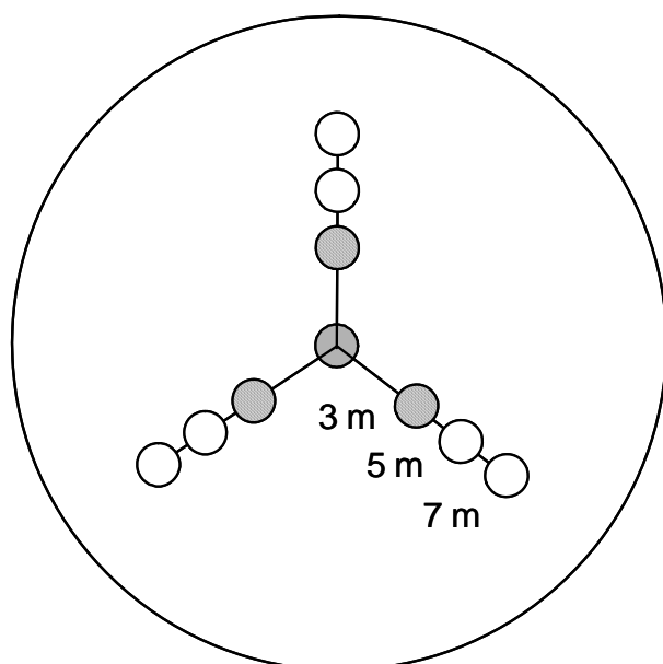
Figur 4.15. Utlägg av småprovytor för kärlväxtregistrering i ängs- och betesmarksobjekt. I de tre inre småprovytorerna (skuggade) görs NILS småprovytemetodik som vanligt, och i alla nio görs registrering av ängs- och betesmarksarterna.
