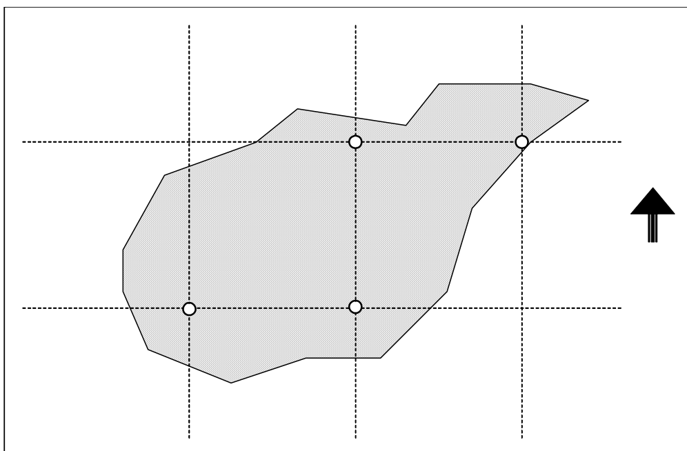
Figur 4.5. Exempel på provyteutlägg i ängs- och betesmarksobjekt. Koordinaterna har tagits fram utifrån ett jämnt ruttmönster med slumpad startpunkt.
