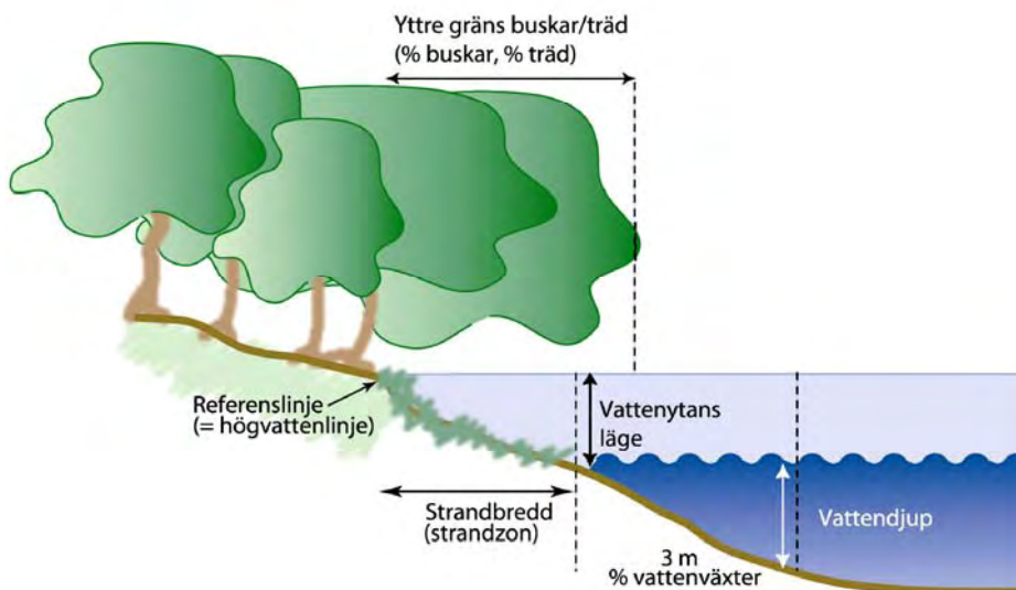
Figur 6.8. Referenslinje, zoner och storleksmått vid stränder.
