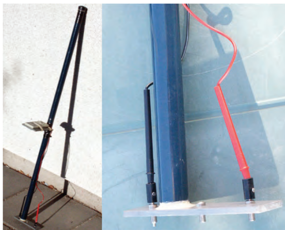
Figur 4.12. Mätsond (kalibreringsstav) med 5 respektive 10 cm avstånd (olika fisklängder) mellan elektroderna för att mäta spänningsgradienten omkring elektroderna och kontrollera utrustningen.
