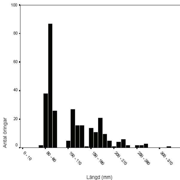
Figur 10.1. Längdfördelning för öringungar i ett strömlevande bestånd i Västra Dalkarlsån, Västerbotten.
