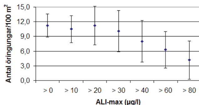
Figur 13.8. Genomsnittlig täthet (antal/100 m²) av öringar i relation till högsta uppmätta halt av oorganiskt aluminium (ALI_max) i IKEU-vattendragen 1998-2006. Felstaplarna visar +/- 2 SE (standard error) (Bergquist & Dahlberg 2009).
