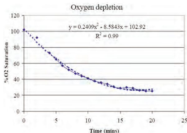
Figur 9.5. Syrgastärning i hink med 45 liter vatten och regnbåge utgörande 50 % av vattenvolymen. Vattentemperaturen är 14° C (från Beaumont m.fl. 2002).
