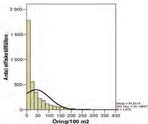
Figur 12.1. Beräknad täthet av insjööring (hela Sverige). Enstaka värden upp till 700 är inte redovisade. Normalfördelningskurva är inlagd.
