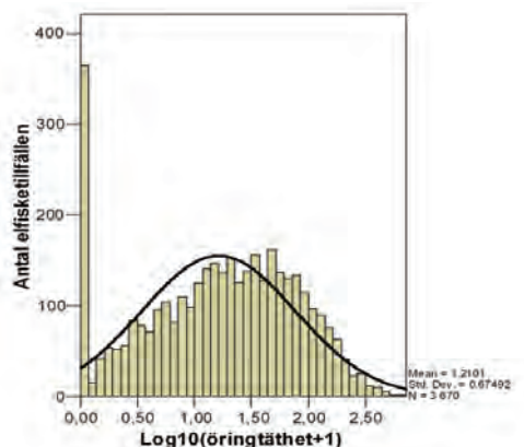
Figur 12.2. Samma data som i figur 11.1, men transformerade med \log_{10}(\text{öringtäthet}+1) .
