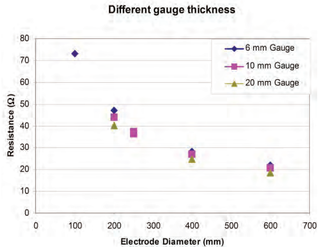
Figur 4.13. Ekvivalenta elektrodresistanser för olika anodringar vid en konduktivitet av 35 mS/m (från Beaumont m.fl. 2005).
