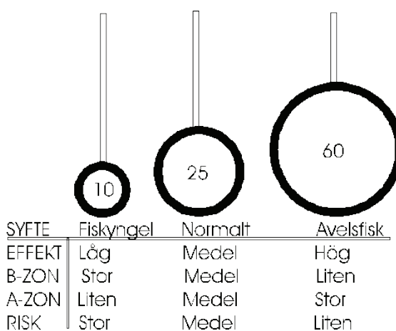
Figur 5.3. Lämplig diameter (cm) på anodringen utgående från storlek på fisken. B-zon är bedövningszon och A-zon är attraktionszon.
