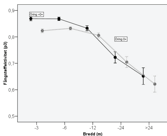
Figur 5.8. Fångsteffektivitet för öring avsett mot vattendragets bredd efter tre utfisken ( p_3 ) i medeltal för inrapporterade elfisken till SERS. Fångsteffektiviteten visar hur stor andel av den totala populationen som skattas ha fångats efter tre utfisken.
