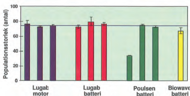
Figur 5.10. Skattad populationsstorlek för ettårig Gullspångsöring (medellängd 153 mm) med 95 % konfidenstervall vid fiske med olika typer av elfiskeaggregat och en temperatur av 10,6 - 12,2 °C. Helt dragen linje anger faktiskt antal öringindivider (från Näslund 1996).
