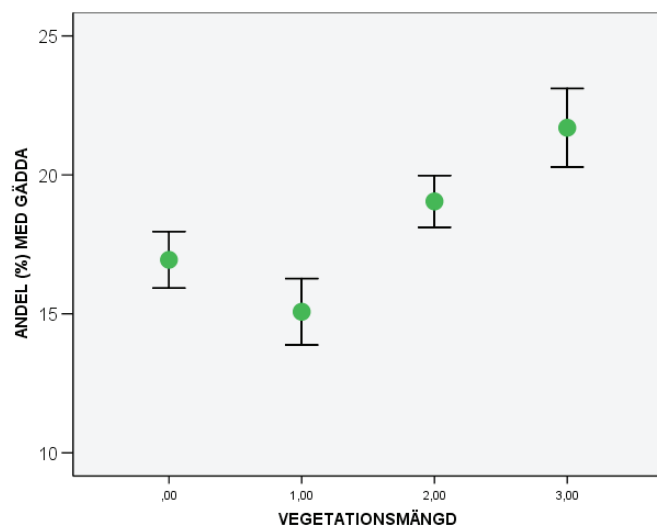
Figur 13.4. Andel (%) elfiskelokaler med förekomst av gädda i relation till vegetationsmängden (klassad 0-1-2-3) på lokalen.
