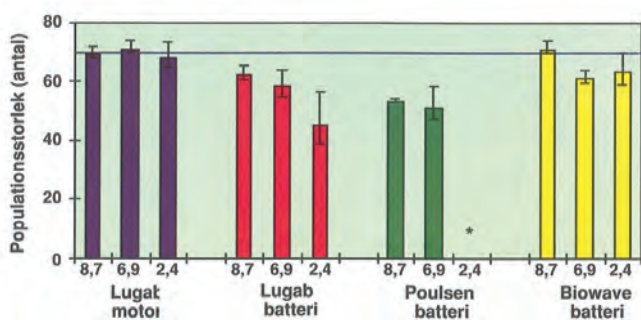
Figur 5.9. Skattad populationsstorlek för 0+ öring av Gullspångsstam (medellängd 97 mm) med 95 % konfidenstervall vid fiske med olika typer av elfiskeaggregat vid tre olika temperaturer 8,7 och 6,9 samt 2,4 °C. Aggregaten var Lug AB motor (L 1000) och batteri (Lug-puls, 50 Hz), Poulsen batteri (Pou-puls, 70 Hz) samt Biowave batteri (Biow-puls, 400 Hz). Helt dragen linje anger faktiskt antal öringindivider (från Näslund 1996).
