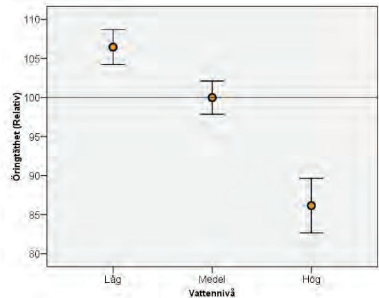
Figur 5.7. Normerad öringtäthet (100 = normal) per lokal avsatt mot vattennivån vid elfisketillfället (kustvattendrag med lång uppföljning) (från Degerman m.fl. 2010).
