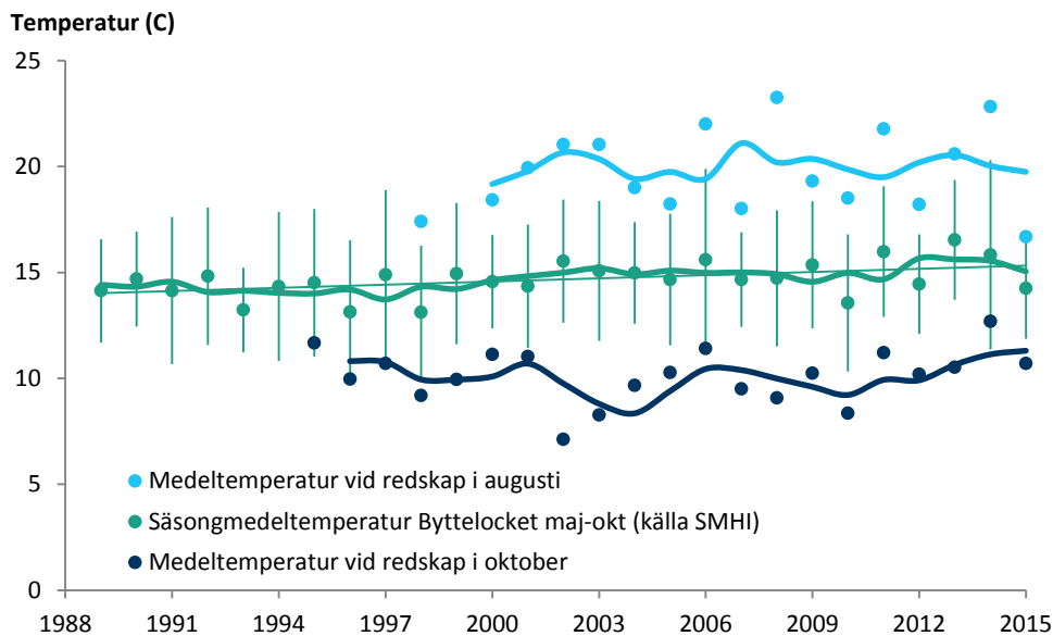
Figur 2. Temperaturer vid redskap vid provfiske i augusti och oktober samt säsongstemperaturen under maj till oktober vid fem meters djup (Byttelocket, källa SMHI). Vertikala linjer anger 95 % konfidensintervall. De grövre linjerna visar tre års glidande medelvärde. Tunn linje visar signifikant trend. Notera att data från åren 2013 och 2014 visar medelvärdena för säsongstemperaturen i Byttelocket baserade på juli-oktober (2013) respektive maj-augusti (2014).
