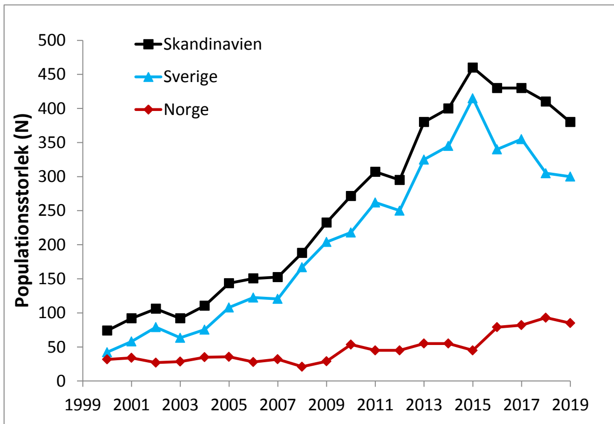
Figur 1. Populationsutveckling av varg under perioden 1999 till 2019 för den skandinaviska populationen (svart), den svenska delpopulationen (blå) samt den norska delpopulationen (röd). Populationsstorleken per 1 oktober för respektive år är angiven som bruttopopulation ( N_{\text{brutto}} ) vilket inkluderar funna levande och döda vargar under inventeringssäsongen (1/10–30/3). Populationsskattningarna är hämtade från de årliga nationella statusrapporterna som produceras av Viltskadecenter (Sverige) och Rovdata (Norge).
