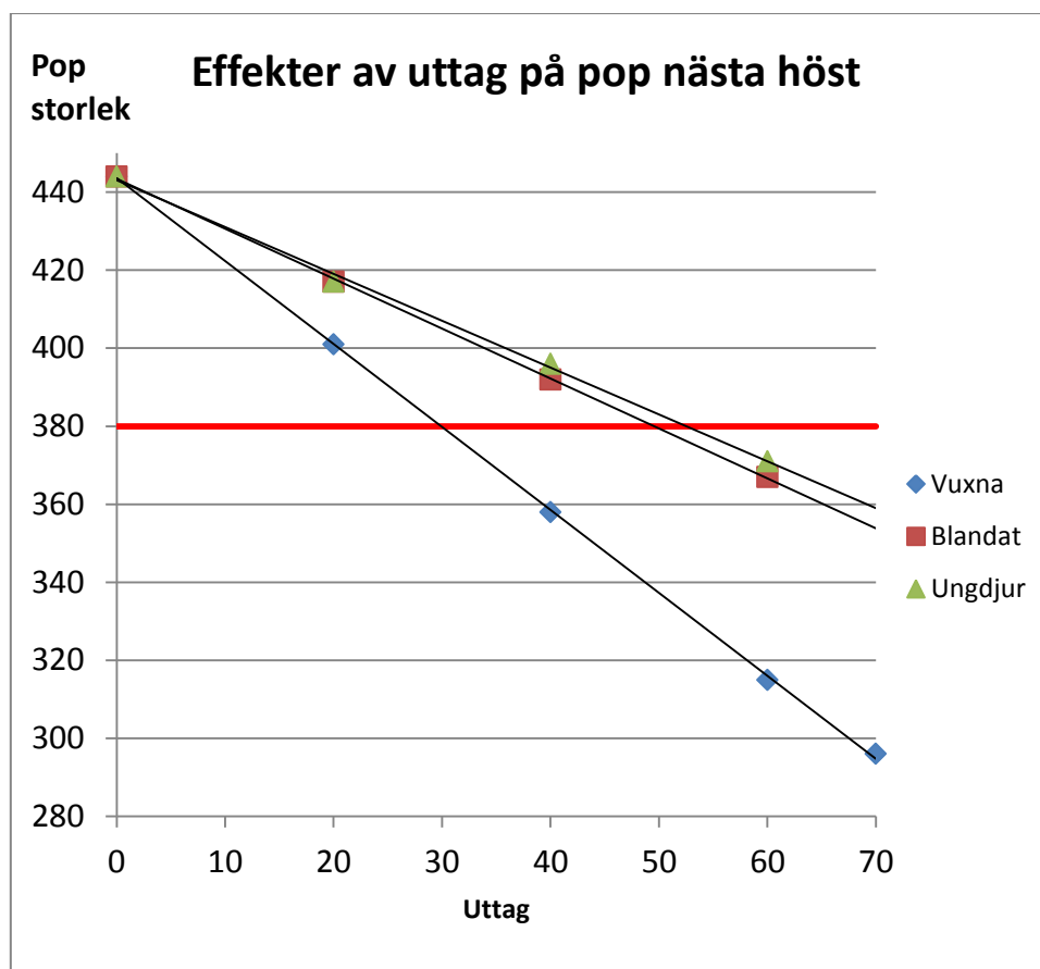
Figur 4. Effekter av tre olika jaktstrategier under jakten 1 maj 2019 - 30 april 2020 på hur stor populationen blir hösten 2020. Nivån för bruttopopulationen hösten 2018 på 380 vargar är markerad i figuren med röd heldragen linje.
