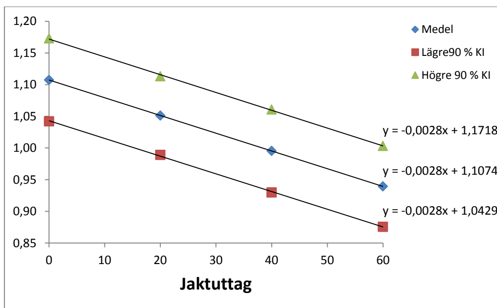
Figur 3. Sambandet mellan jaktuttag 2019/2020 och den resulterande tillväxten i den skandinaviska populationen från vinter 2019 till vinter 2020. Den översta och understa linjen visar gränserna för 90% konfidensintervall.
