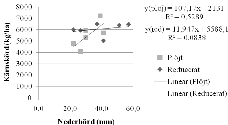
Figur 25. Kärnsköörden som funktion av sammanlagd nederbörd under 1 månad efter sådd.
