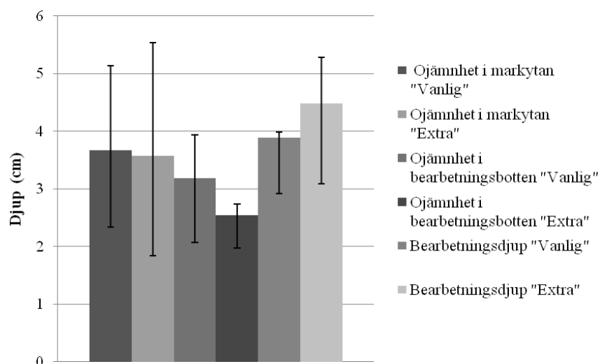
Figur 30. Medelvärden av ojämnhet i markytan 1, ojämnhet i bearbetningsbotten 2, samt bearbetningsdjupet 3 för vanlig respektive extra harvning.
