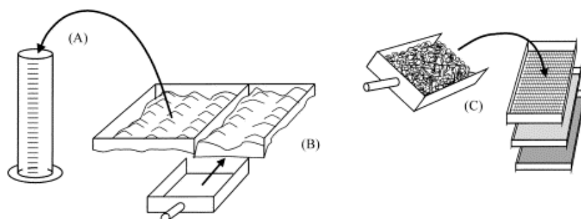
Figur 10. Hur såbäddsundersökningen fungerar i fält. Mätcylinder (A), Stålram (B) och skiktscopa (C) Efter Håkansson (2002).
