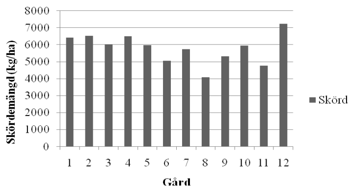
Figur 18. Gårdarnas kärnskörd i kg/ha för plöjningsfria system (1-6) och plöjda system (7-12).
