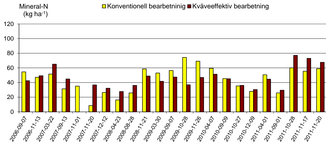
Figur 7. Mineralkväve i marken, 0-90 cm djup, i konventionellt och kväveeffektivt system under den andra växtföljdsomgången.
