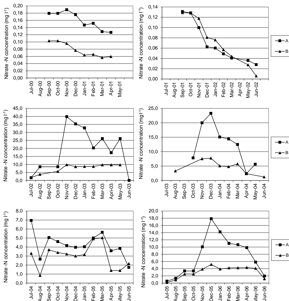
Figur 2. Nitratkoncentrationer (mg l -1 ) i dräneringsvattnet under de hydrologiska åren 00/01-05/06. Månader utan mätvärde saknade avrinning. Observera att skalorna på y-axeln varierar. Led A: Konventionell bearbetning, Led B: Kväveeffektiv bearbetning.
