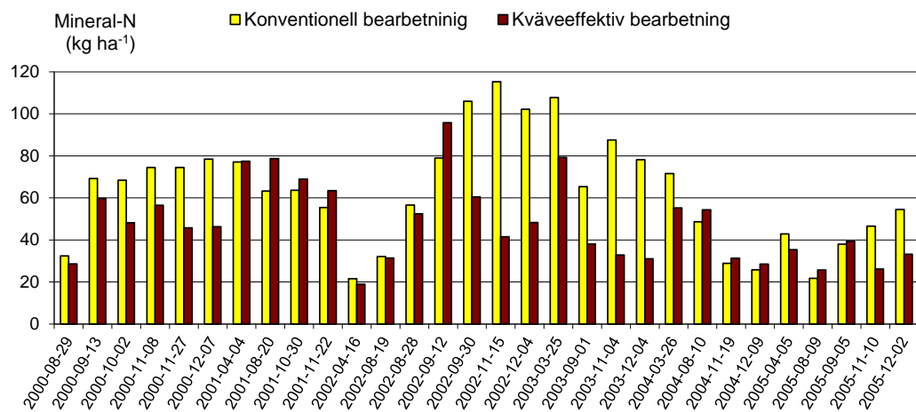
Figur 6. Mineralkväve i marken, 0-90 cm djup, i konventionellt och kväveeffektivt system under den första växtföljdsomgången.
