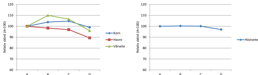
Figur 4.6. Skörd i svenska försök med packning till olika grödor. Vänstra figuren: medeltal av 9 försök. Högra figuren: medeltal av 12 försök. A=inga överfarter, B=en överfart med traktorhjul, lågt ringtryck, C=en överfart, högt ringtryck, D=tre överfarter, högt ringtryck.
