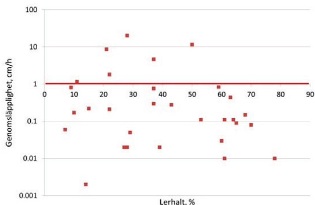
Fig. 4.4. Genomsläpplighet i program för miljöövervakning av markpackning, värden för 30 platser i Sverige som funktion av lerhalt, mätningar 2003-2008. Den horisontella linjen anger 1 cm/h, som ofta anges som gränsvärde för godtagbar genomsläpplighet.
