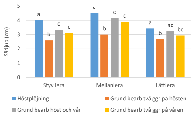
Figur 20. Uppmätt sådjup (cm) i de olika bearbetningsleden. Medeltal av 3 försök på styv lera, 2 på mellanlera och 3 på lättlera. Led inom respektive jordart som ej har samma bokstav är signifikant skilda åt ( p < 0.05 ).
