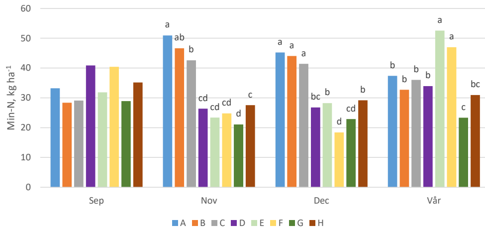
Figur 16. Mineralkväve ( \text{kg N ha}^{-1} ) i marken i 0-90 cm i led A-H i september, november, december och på våren. Medel av fyra försöksår (2012/2013-2015/2016). A=Tidig höstplöjning, med halm, B=Tidig höstplöjning, utan halm, C=Tidig höstplöjning med tältpackare, D=Eftersådd luddvicker/sandhavre, E=Eng rajgräs, höstnedbrukning, F=Eftersådd oljerättika, G=Eng rajgräs, vårnedbrukning, H=Vårplöjning utan fånggröda.
