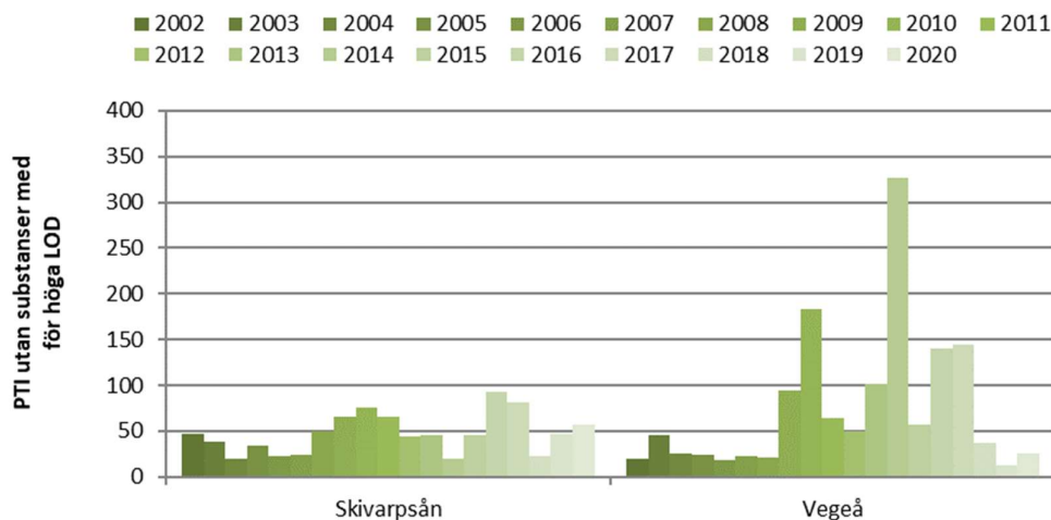
Fig 11b. Toxicitetsindex (PTI) beräknat för två Skånska åar, 2002-2020, men där substanser med för höga detektionsgränser i förhållande till riktvärden inte inkluderats, se Tabell 1.
