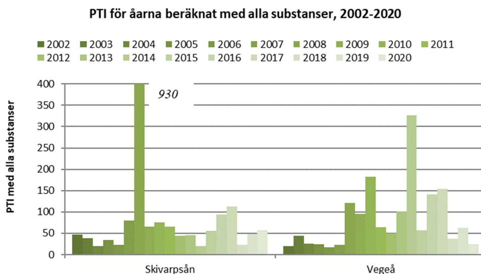
Fig 11a. Toxicitetsindex (PTI) beräknat för två Skånska åar, 2002-2020, med alla analyserade substanser.
