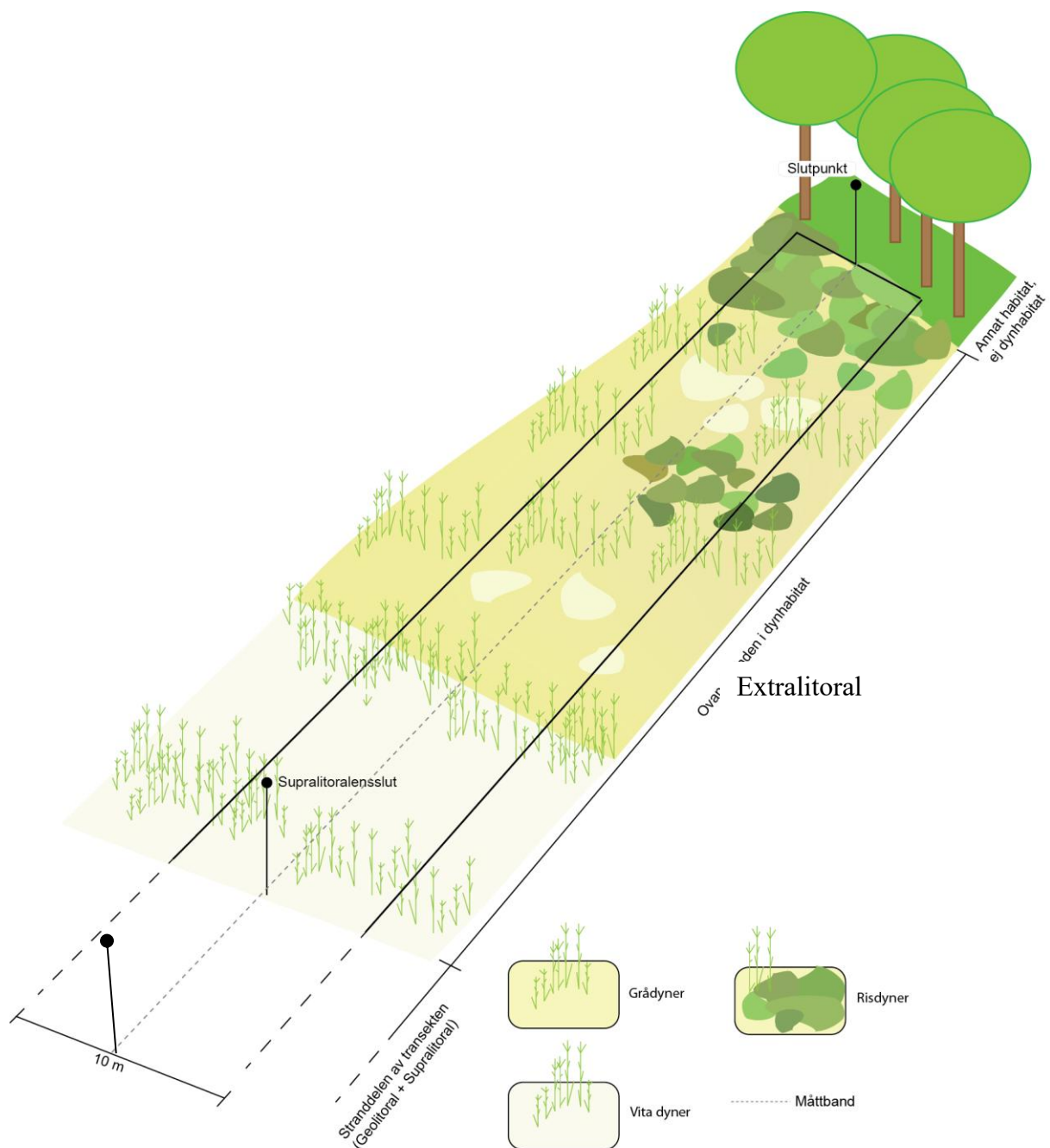
Figur 5. Transekt som visar hur dyngabitaten kan avlösa varandra inom transektens extralitoral. Fördelningen mellan de olika dyngabitaten anges som den sträcka längs måttbandet (transektens mittlinje) som träffar resp. typ. Blottad sand inom dyngområdet mäts på samma sätt. Transektens slutpunkt sätts där dyngområdet slutar (i detta fall i en skog som inte klassas till 2180 Trädklädda dyner).
