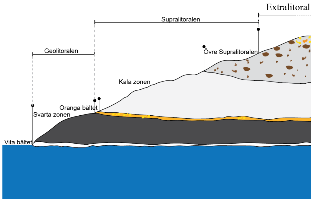
Figur 2. Skiss av en häll/klippstrand. Geolitoralerna består längst ned av en zon som domineras av havstulpaner, s.k. vita bältet, följt av en zon dominerad av antingen cyanobakterier (s.l. såpor, sl. Calothrix ) eller svartlav ( Verrucaria maura ) den s.k. svarta zonen. Supralitoralerna består längst ned av en zon dominerad av orangelavar (sl. Caloplaca ) det s.k. orangea bältet, följt av den kala zonen som i sin tur följs av ett område med ett välutvecklat lavsamhälle den s.k. "övre supralitoralerna" som är påverkad framför allt av stänk. Extralitoralerna fortsätter till dess klipp/hällarna slutar och annat växtsamhälle tar vid, som inte visar tecken på att vara påverkad av aerosoler.
