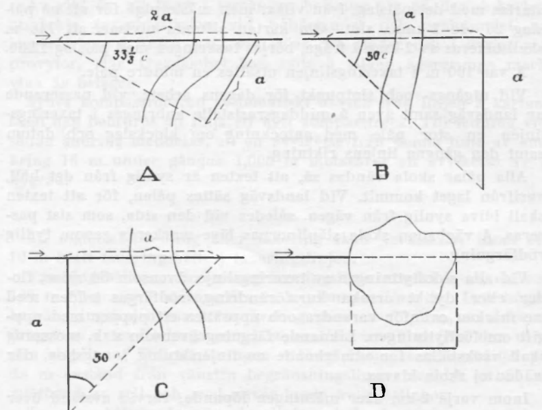
Fig. 1. Tillvägagångssätt vid mätning av vattendrag. Heldragna linjer ange sträckor, som uppmätas. (D utvisar vinkling).
