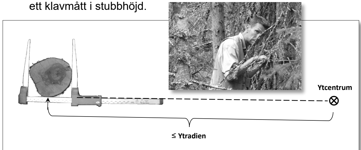
Fig. 7.2 Klaven ska hållas vinkelrätt mot trädets längdaxel och med linjalen riktad mot provytans centrum.
