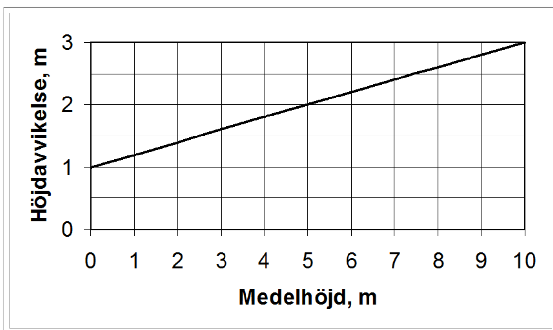
Fig. 5.7 Minimikrav på höjdavvikelse mellan två skikt där medelhöjden för det högsta skiktet är lägre än 10 m.
