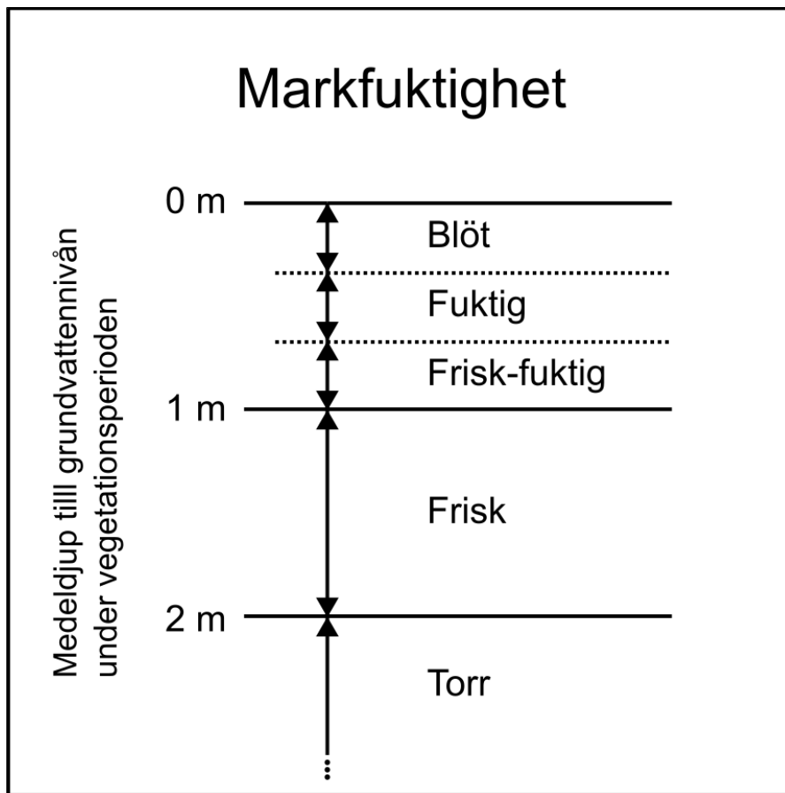
Fig. 11.6.4.1 Förenklad skiss. Markfuktigheten bedöms i första hand genom att grovt skatta djupet ned till grundvattentytans genomsnittliga nivå under vegetationsperioden. Detta djup varierar säsongs- och årsvis.
