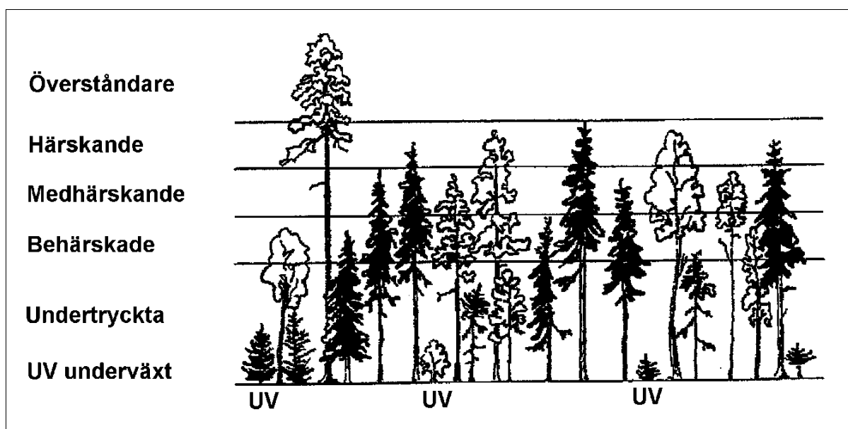
Fig. 8.1 Trädklasser.
