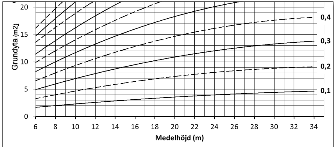
Fig 6.3 Diagram för bestämning av preliminär massaslutenhet
