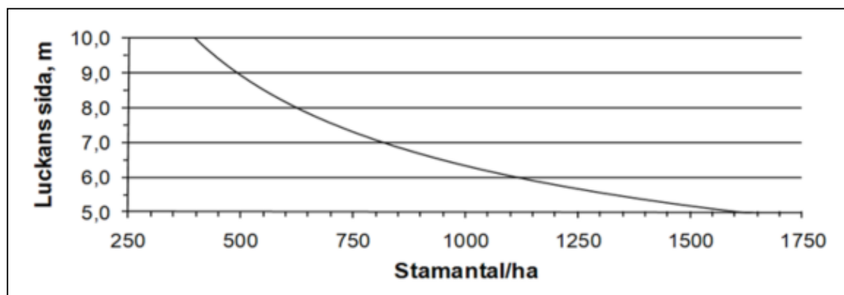
Fig. B.2.4 Sambandet mellan stamantal och luckans sida
