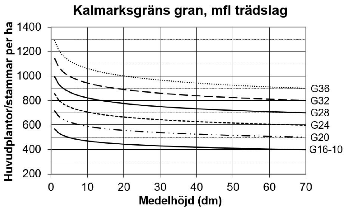
Fig. 6.2 Diagram för bestämning av kalmarksgräns för gran, mfl trädslag
