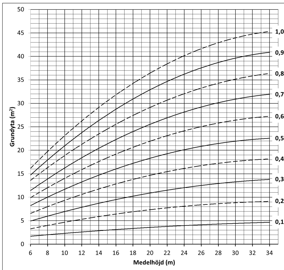
Fig. B.2.3 Preliminär massaslutenhet.
