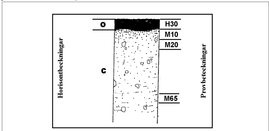
Fig. 11.6.23.8 Horisont- och provbeteckningar – Regosol (exempel).
