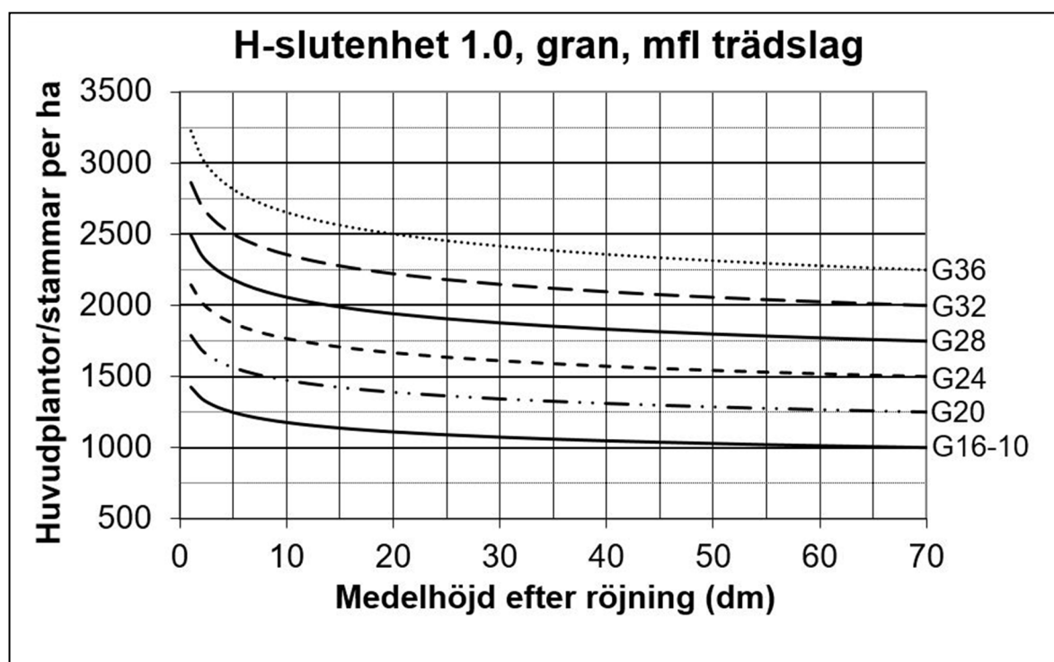
Fig. B.2.2 Krav för H-slutenhet 1.0 – gran, m.fl. trädslag.
