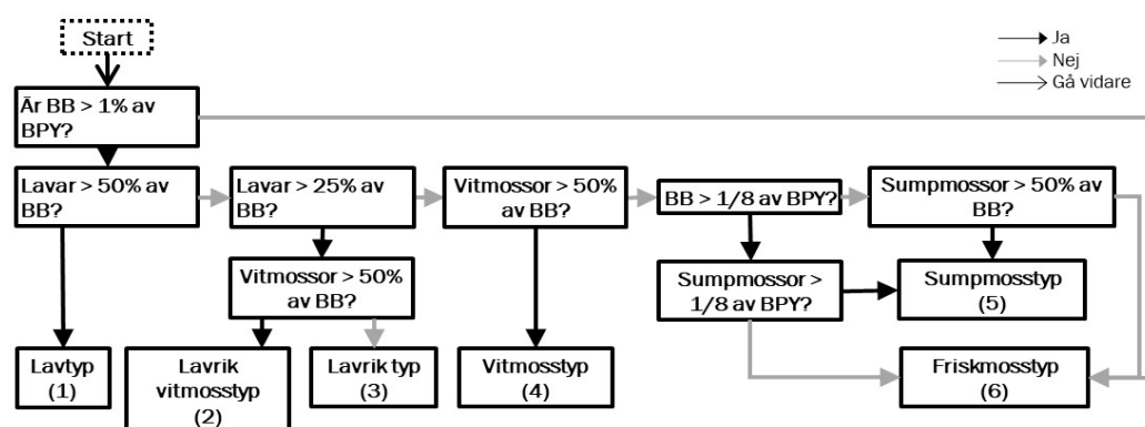
Fig. 5.2 Schema för klassning av bottenskikt.
