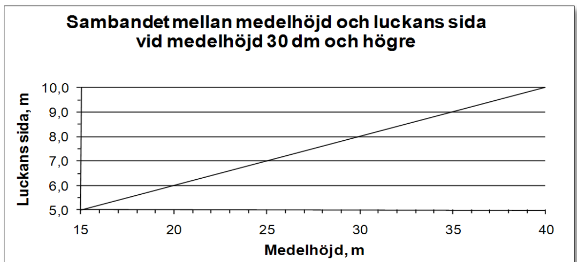
Fig. B.2.5 Samband mellan medelhöjd och luckans sida vid medelhöjd 30 dm och högre
